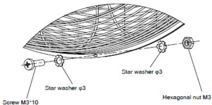
Abb.5-7: Sicherung der Schutzkörbe montieren
