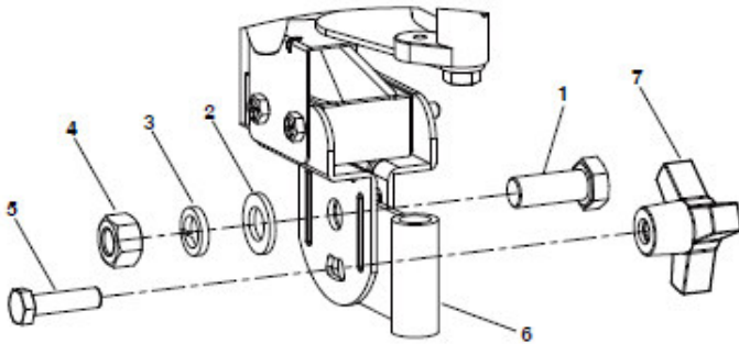
Abb. 5-8: Montage des Gelenkstücks
