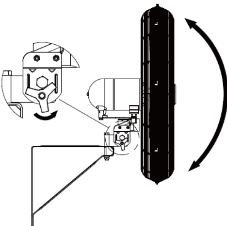
Abb. 5-10: Einstellung des Neigungswinkels
