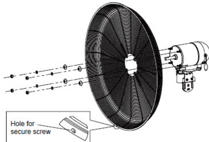
Abb.5-4: Montage des hinteren Schutzkorbs
