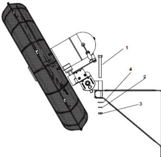
Abb. 5-9: Montage des Ventilatorkopfs an die Wandhalterung
