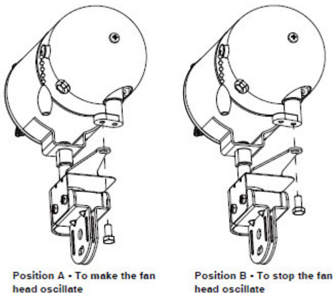
Abb. 6-1: Oszillationsfunktion
