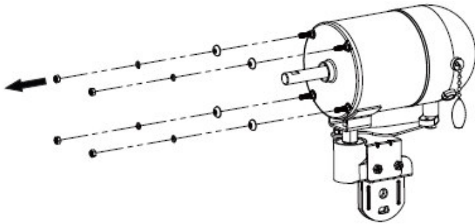
Abb.5-3: Befestigungselemente vom Motor entfernen
