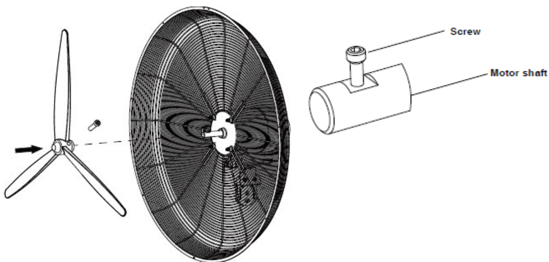
Abb.5-5: Montage des Lüfterrads
