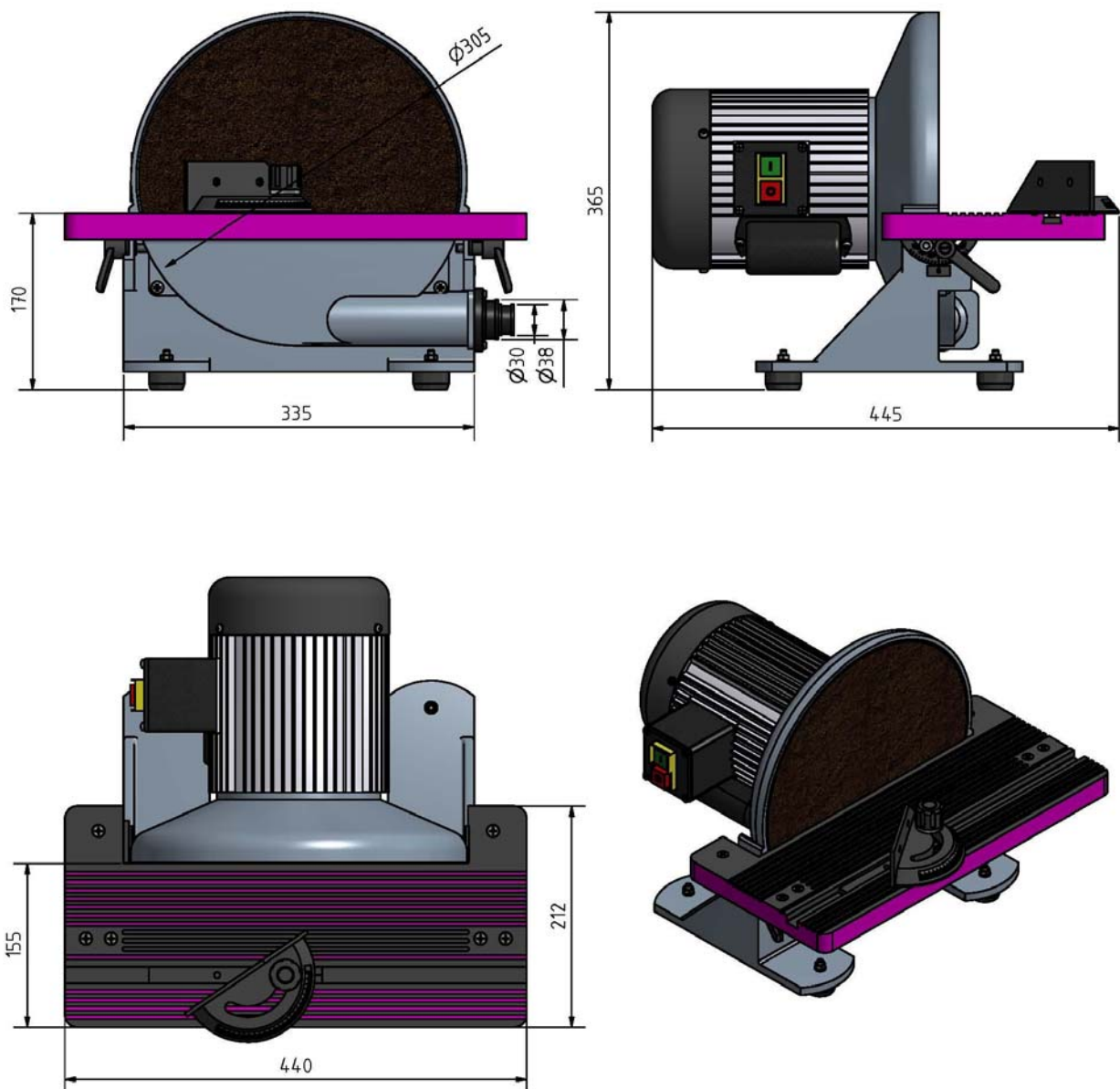
Abb.2-1: Abmessungen
