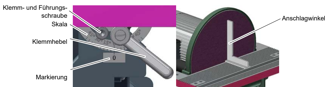
Abb.4-3: Winkel einstellen
