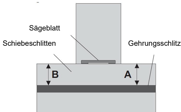
Abb. 53: Schiebeschlitten ausrichten
