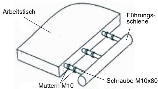
Abb. 12: Anschlag-Führungsschiene montieren
