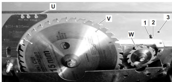
Abb. 7: Sägevorrichtung
