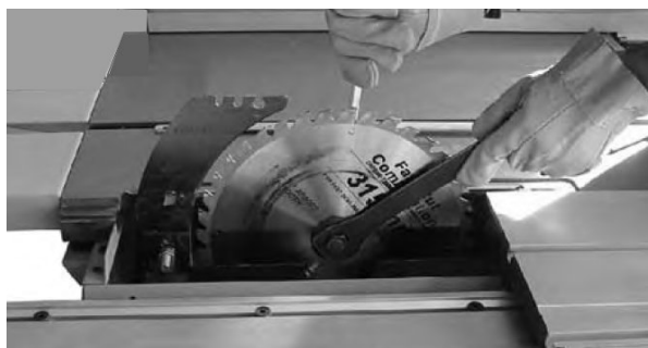
Abb. 45: Sägeblatt abschrauben
