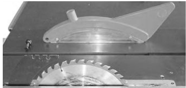
Abb. 24: Sägeblattschutz montieren
