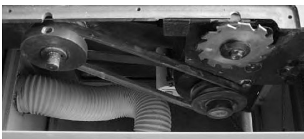
Abb. 50: Antriebsriemen austauschen
