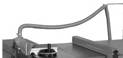
Abb. 26: Absaugschläuche montieren
