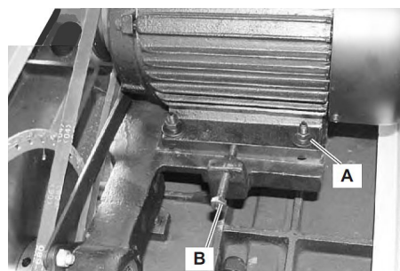
Abb. 51: Motorschrauben lösen
