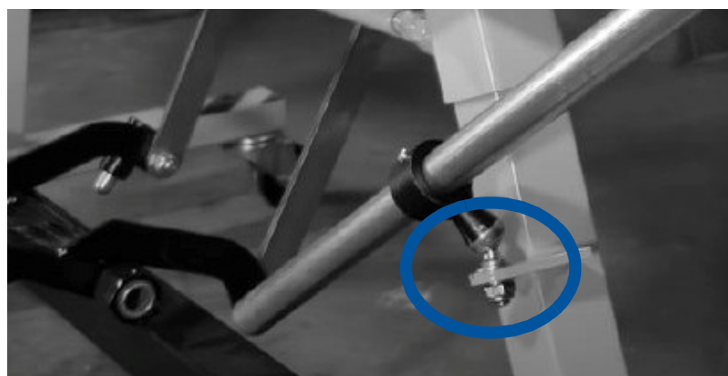
Abb.6-14: Montage Unterseite Gasfeder
