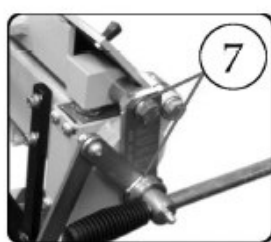
Verbindungen des Hebemechanismus der Oberwange
