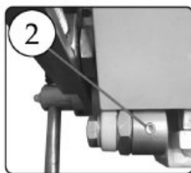
Welle des Biegewangenscharniers
