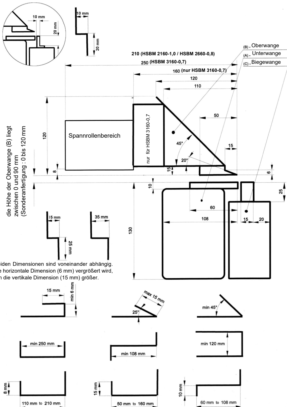
Abb.8-1: Biegeparameter
