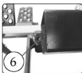
bewegliche Elemente des Pedal-Hebemechanismus der Oberwange
