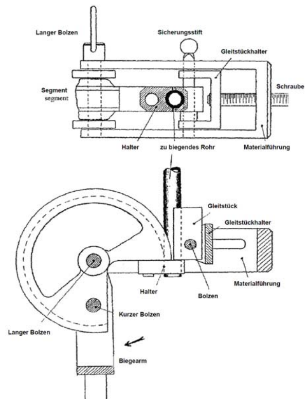
Abb. 2: Aufbau
