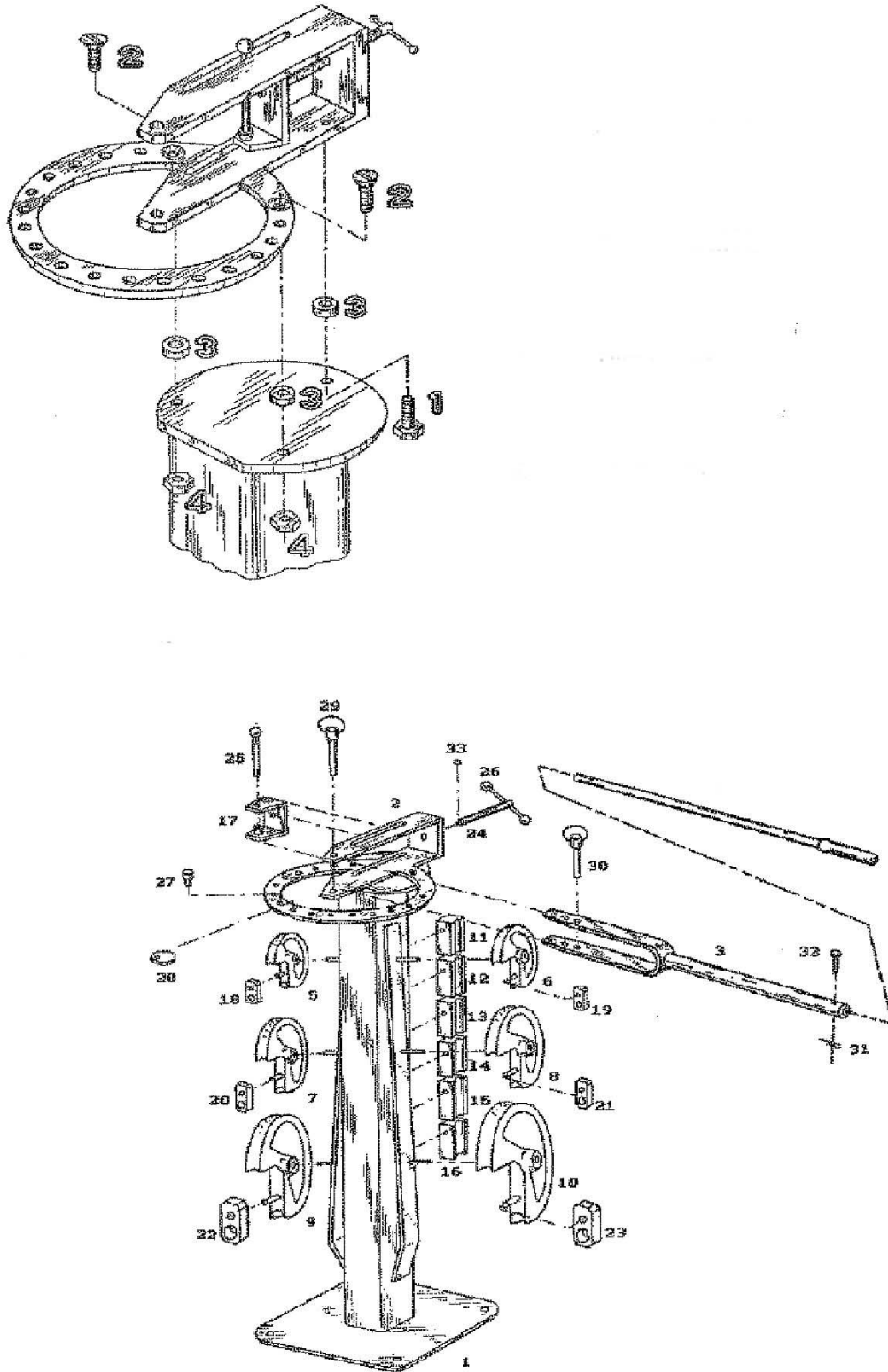
Abb. 4: Ersatzteilzeichnung RB 30
