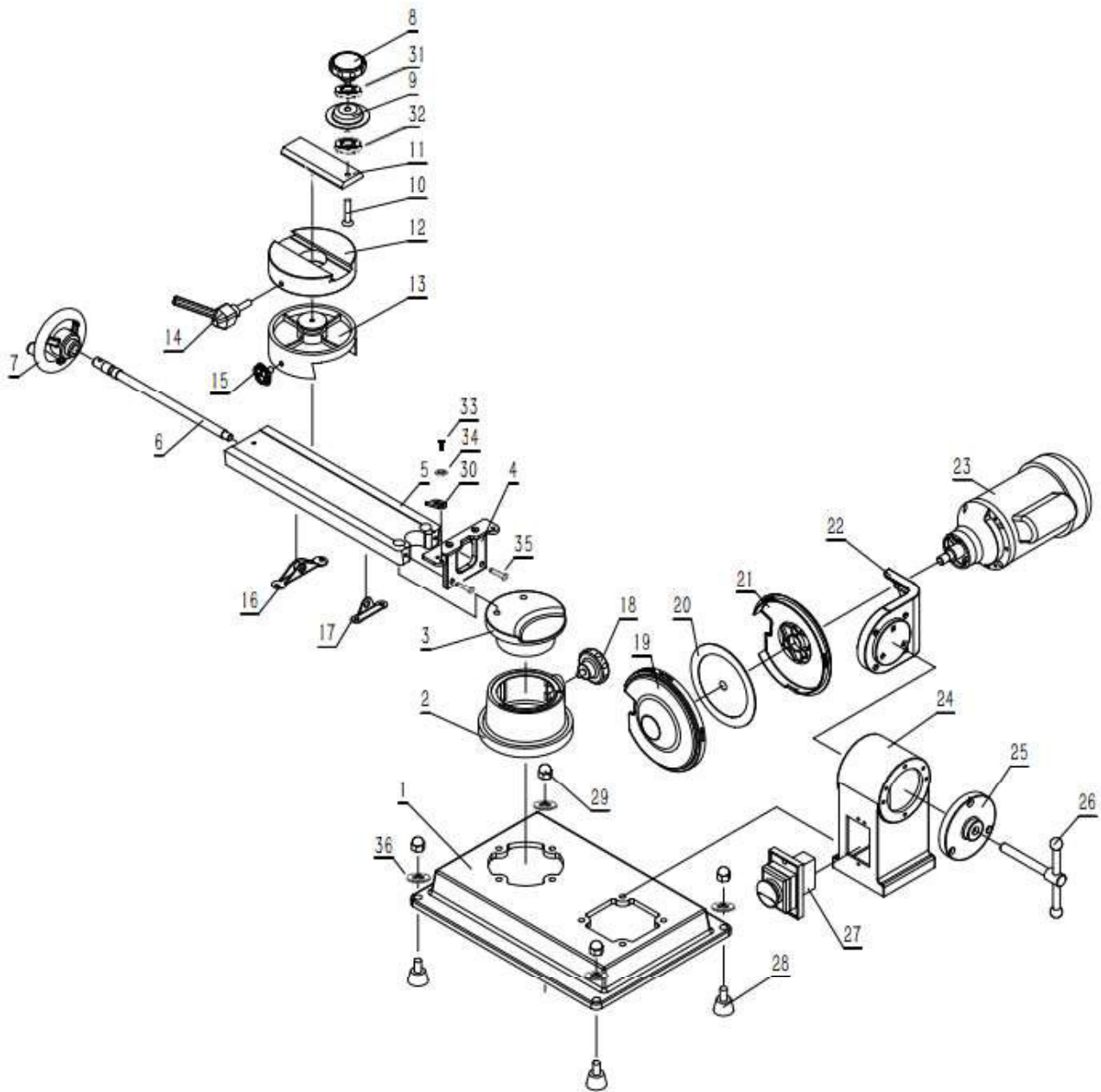
Abb. 9-1: Ersatzteilzeichnung
