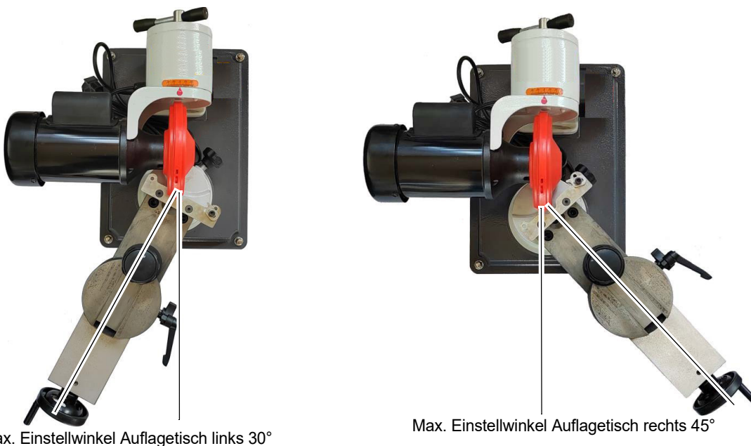
Abb.6-1: Arbeitswinkel einstellen
