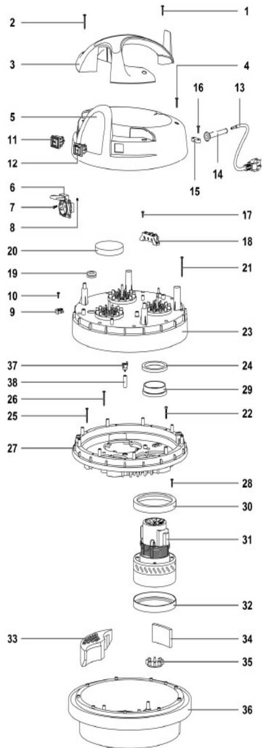
Abb. 10: Ersatzteilzeichnung 1
