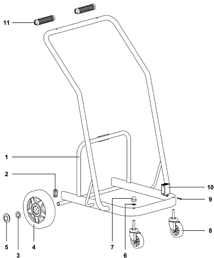
Abb.10 Ersatzteilzeichnung 5 Trockensauger dryCAT 262 RSCT & dryCAT 262 IR SCT
