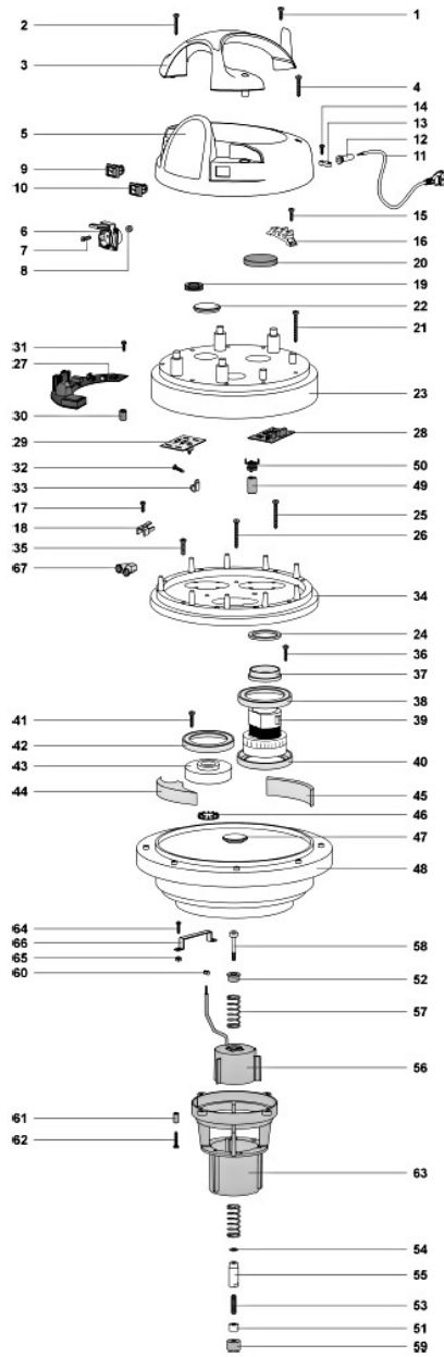
Ersatzteilzeichnung 2 Trockensauger dryCAT 262 RSCT & dryCAT 262 IRSC
