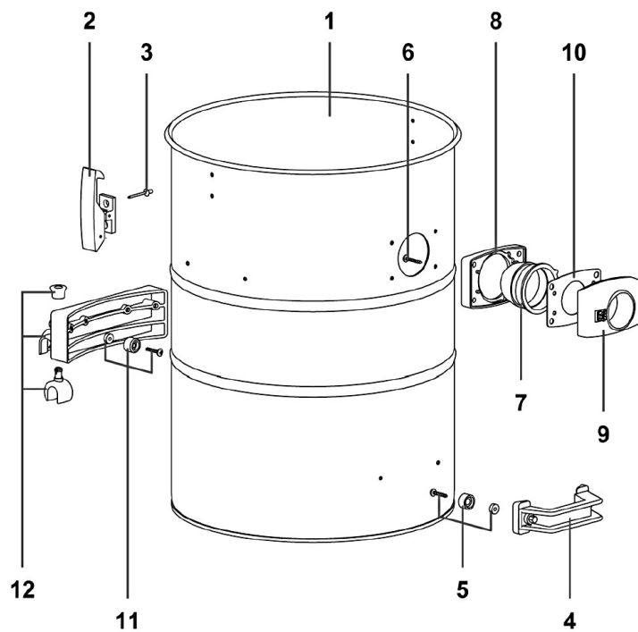
Abb.9 Ersatzteilzeichnung 4 Trockensauger dryCAT 262 IR SCT
