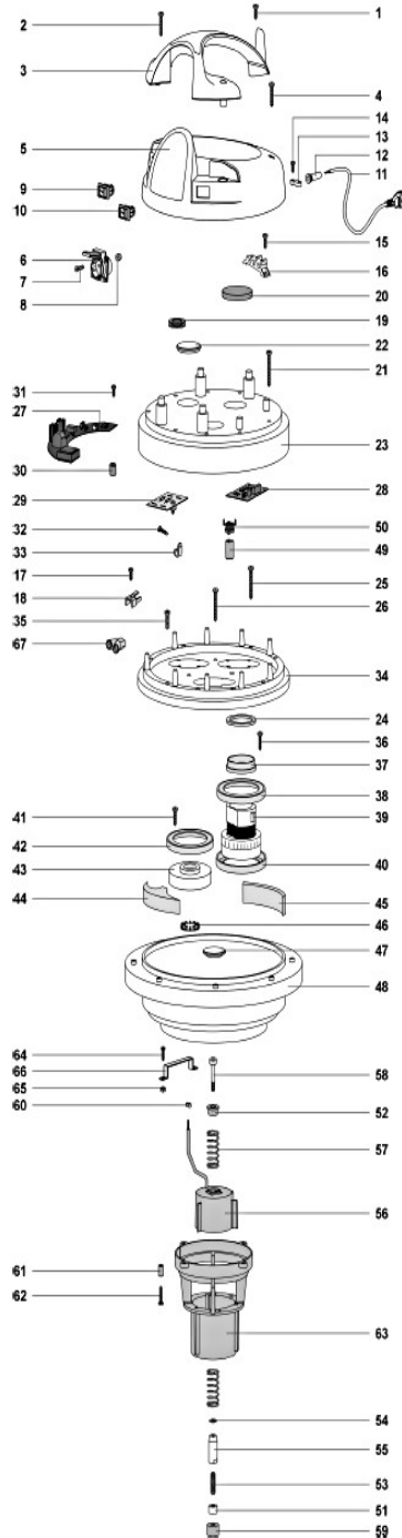
Abb. 7: Ersatzteilzeichnung 1 Trockensauger dryCAT 262 RSCT & dryCAT 262 IRSCT
