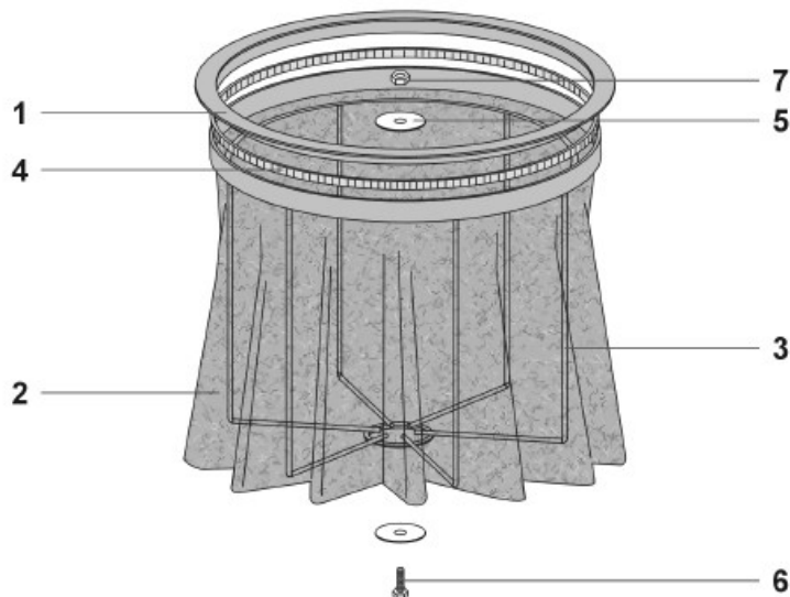
Abb. 8-1: Ersatzteilzeichnungen 1 und 2
