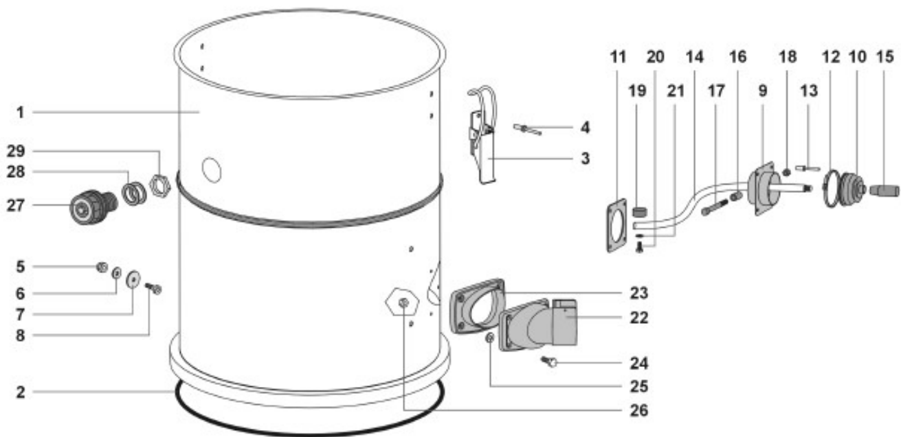
Abb.8-2: Ersatzteilzeichnungen 3 und 4
