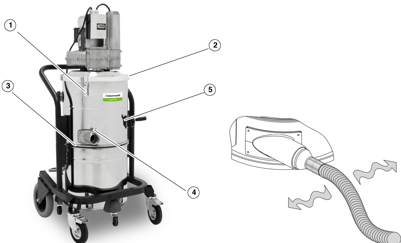
Abb.6-3: Dichtungskontrolle und Saugschlauch
