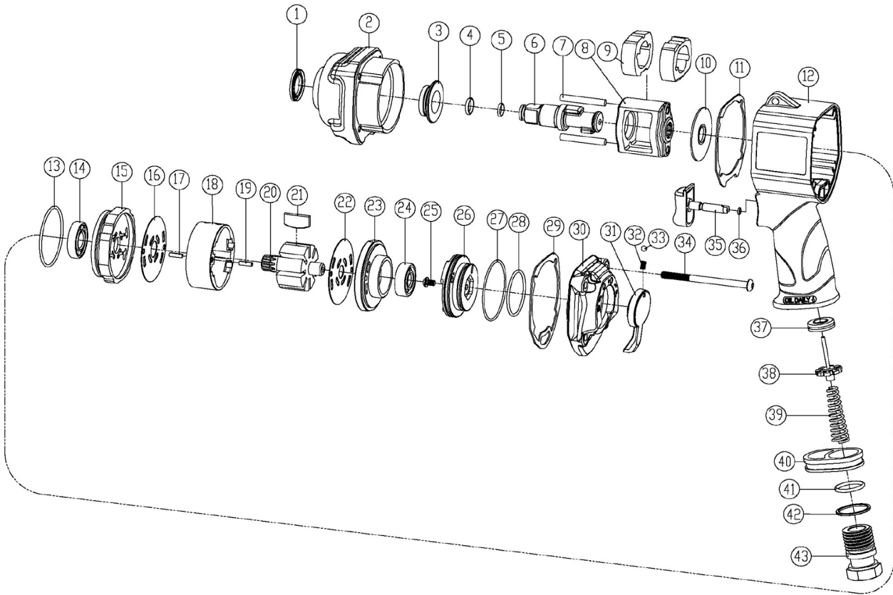
Abb. 3: Ersatzteilzeichnung ISS-TT 1/2" Mini Composite
