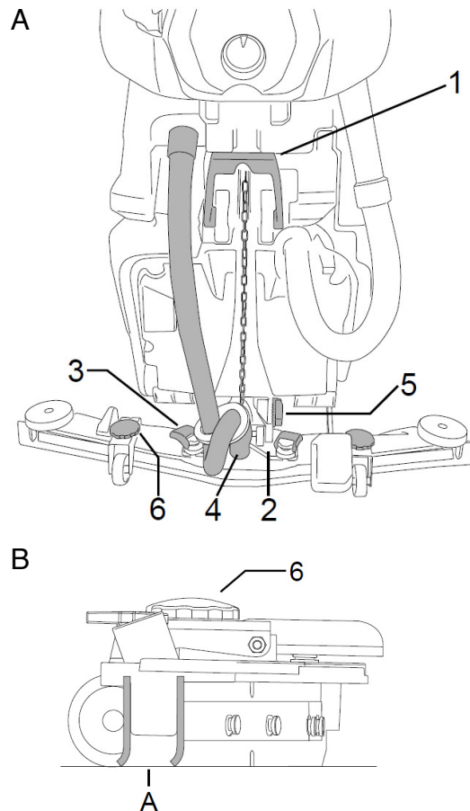
Abb. 9: Montage und Einstellung der Saugleiste
