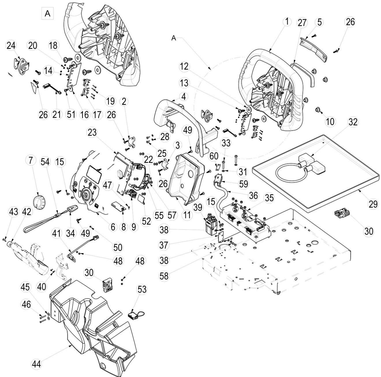
Abb. 56: Ersatzteilzeichnung 15
