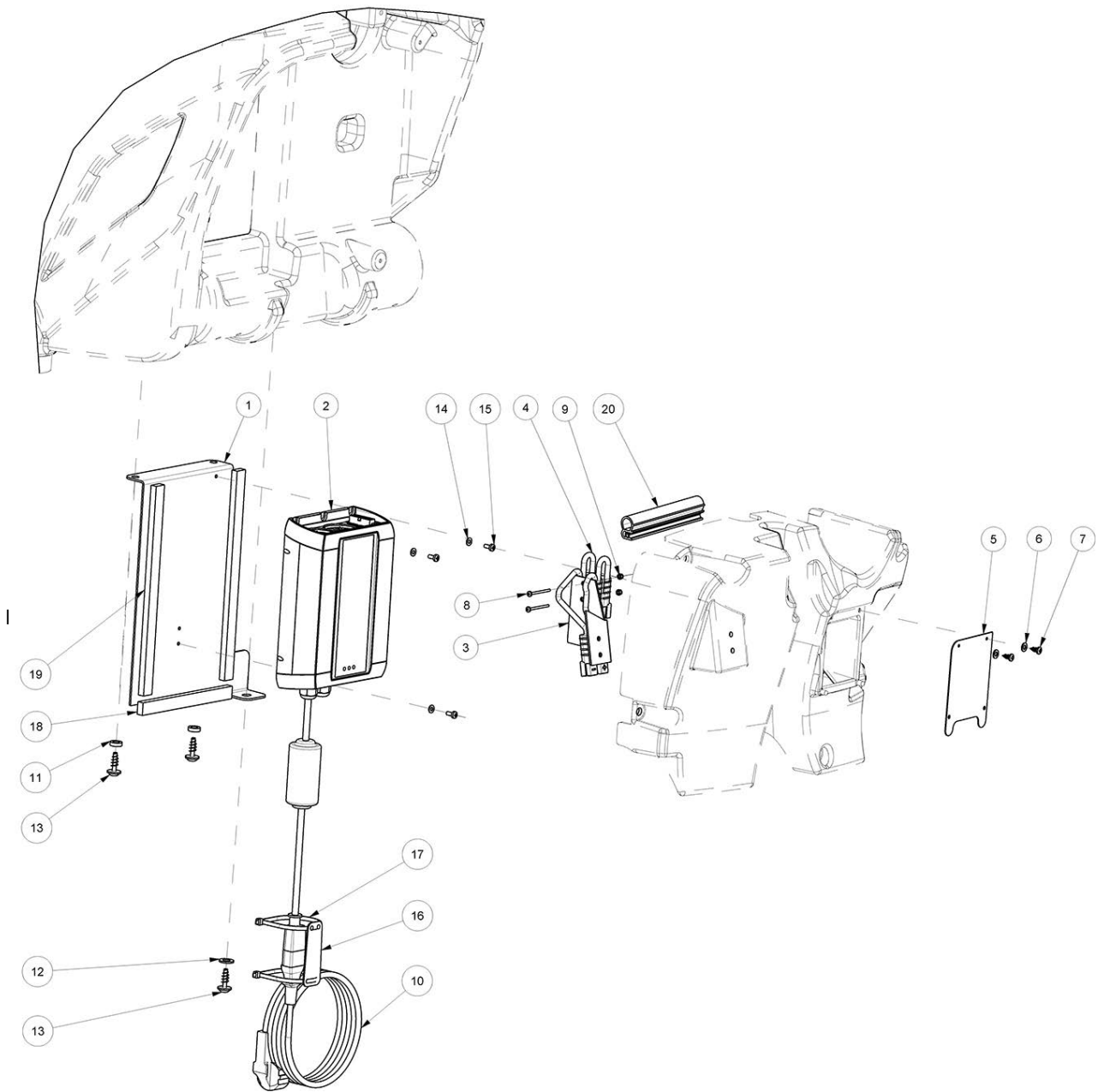
Abb. 52: Ersatzteilzeichnung 9
