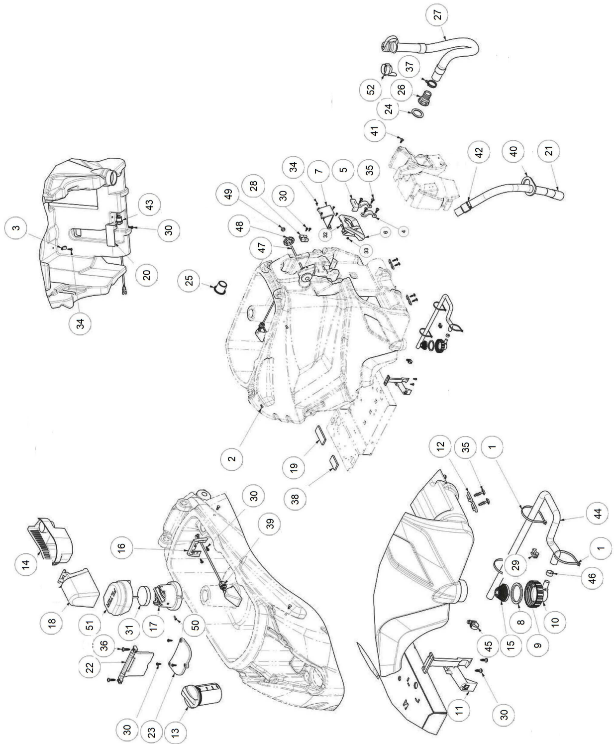
Abb. 27: Ersatzteilzeichnung 7
