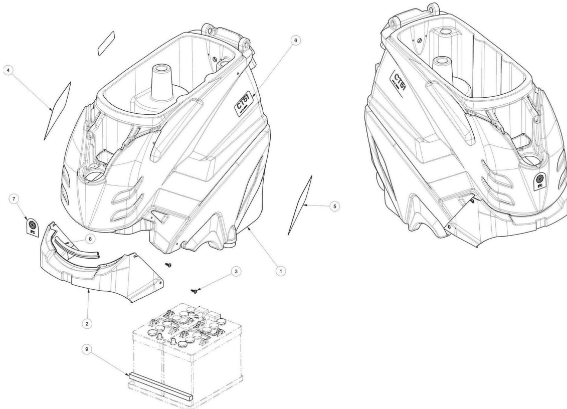
Abb. 40: Ersatzteilzeichnung 9 und Ersatzteilzeichnung 10
