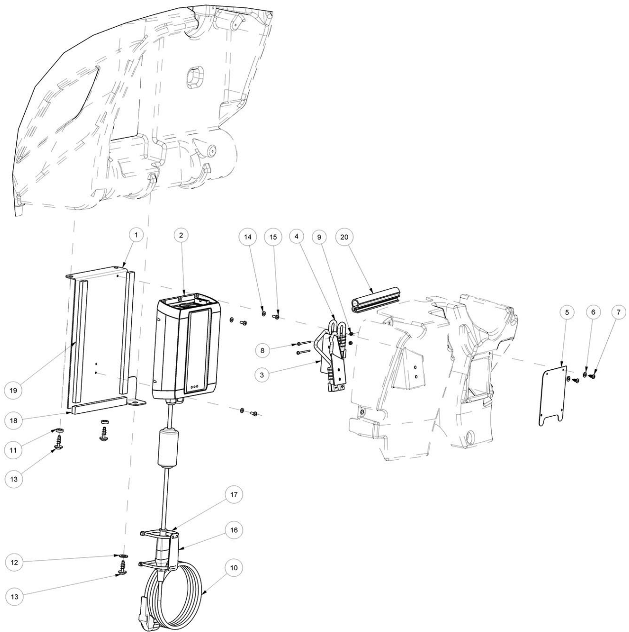
Abb. 41: Ersatzteilzeichnung 11
