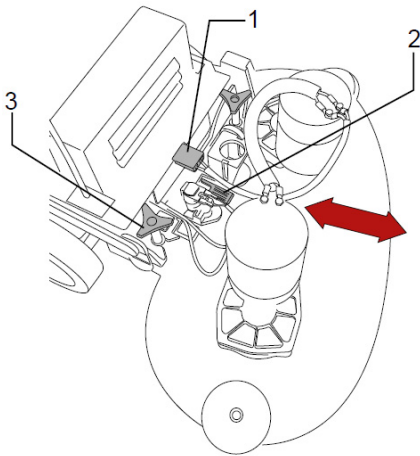
Abb. 12: Schnellwechsel des Reinigungskopfes
