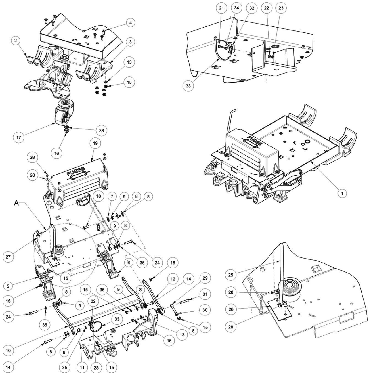
Abb. 44: Ersatzteilzeichnung 14
