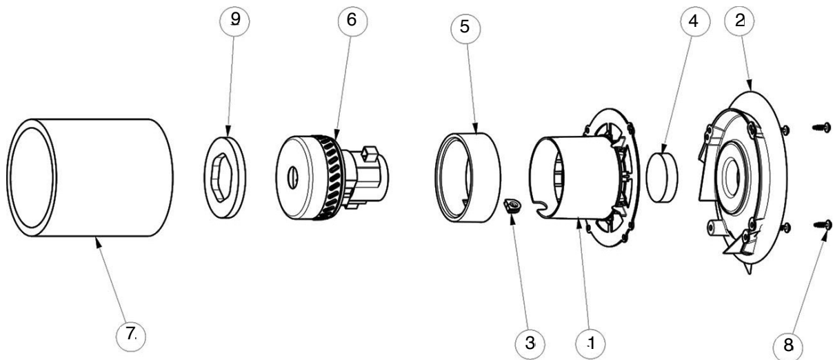
Abb. 35: Ersatzteilzeichnung 3 und Ersatzteilzeichnung 4
