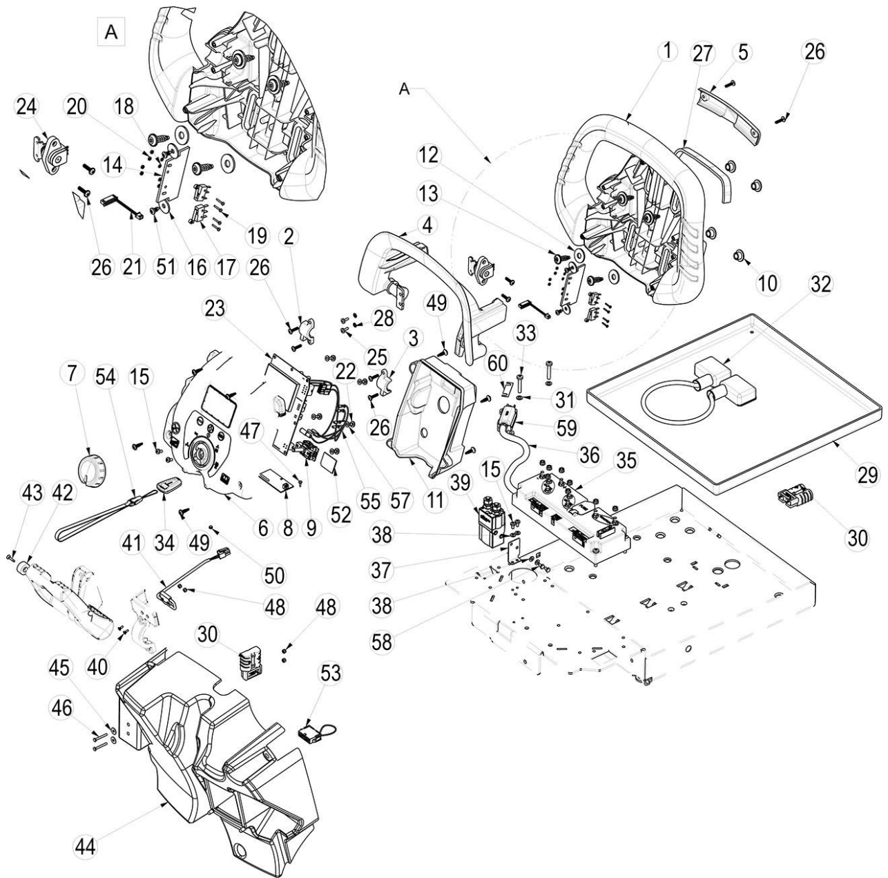
Abb. 25: Ersatzteilzeichnung 4
