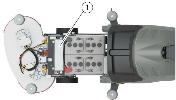
Abb. 18: Auswechseln der Sicherungen
