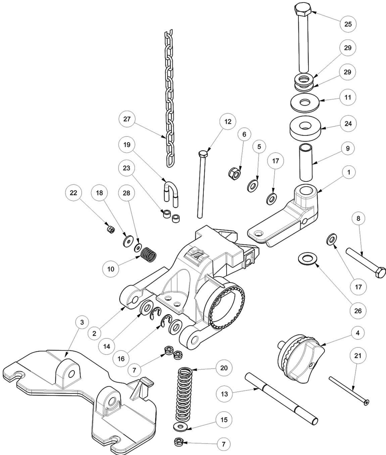
Abb. 22: Ersatzteilzeichnung 1 - Halterung
