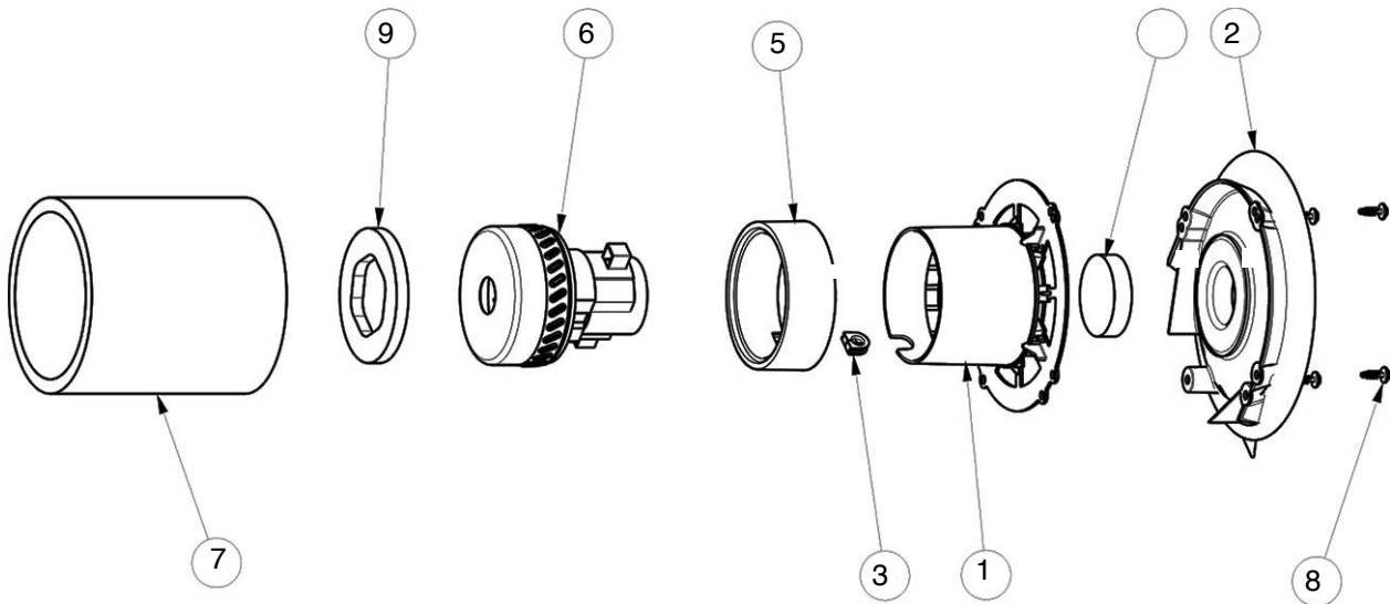
Abb. 26: Ersatzteilzeichnung 5 und Ersatzteilzeichnung 6
