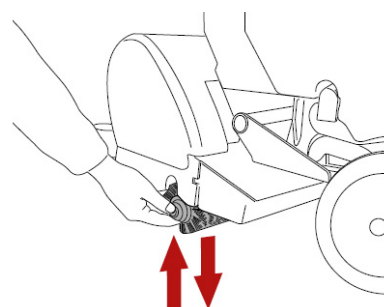
Abb. 11: Anbringen/Freisetzen der Bürstenwalze
