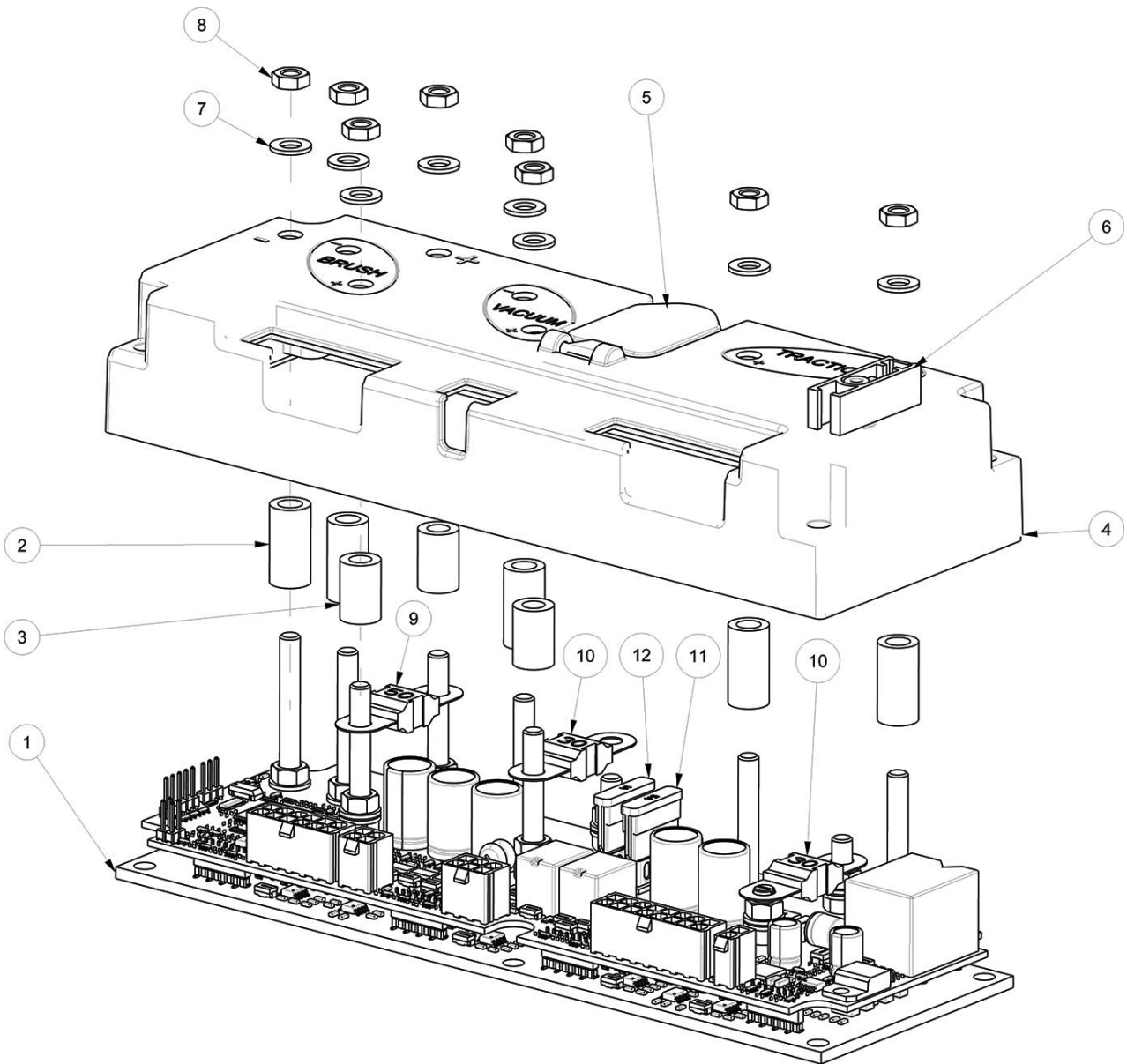
Abb. 42: Ersatzteilzeichnung 12
