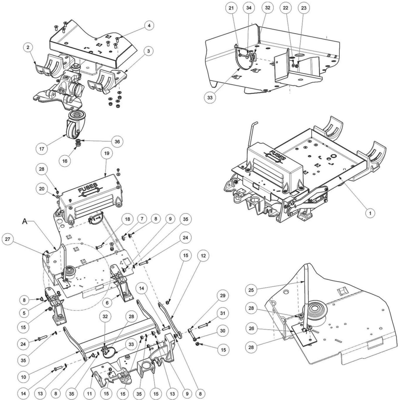
Abb. 46: Ersatzteilzeichnung 1
