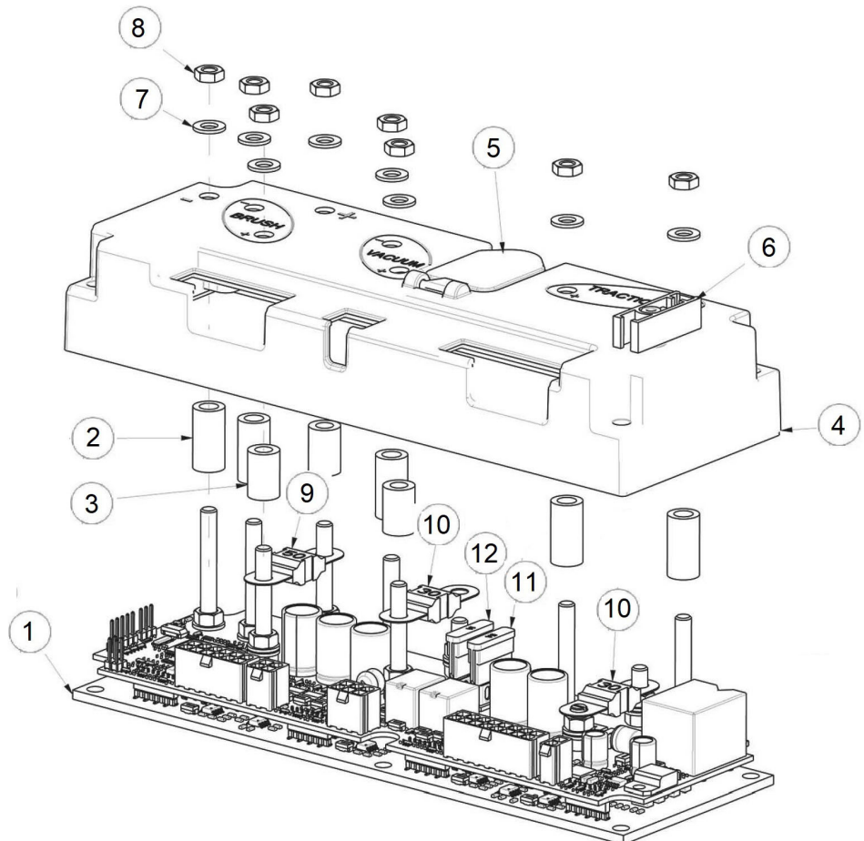
Abb. 29: Ersatzteilzeichnung 10 und Ersatzteilzeichnung 11
