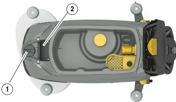
Abb. 16: Wasser-/Reinigungsmittel-tank
