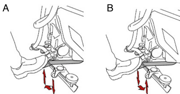
Abb. 10: Automatisches Einhängen der Bürste
