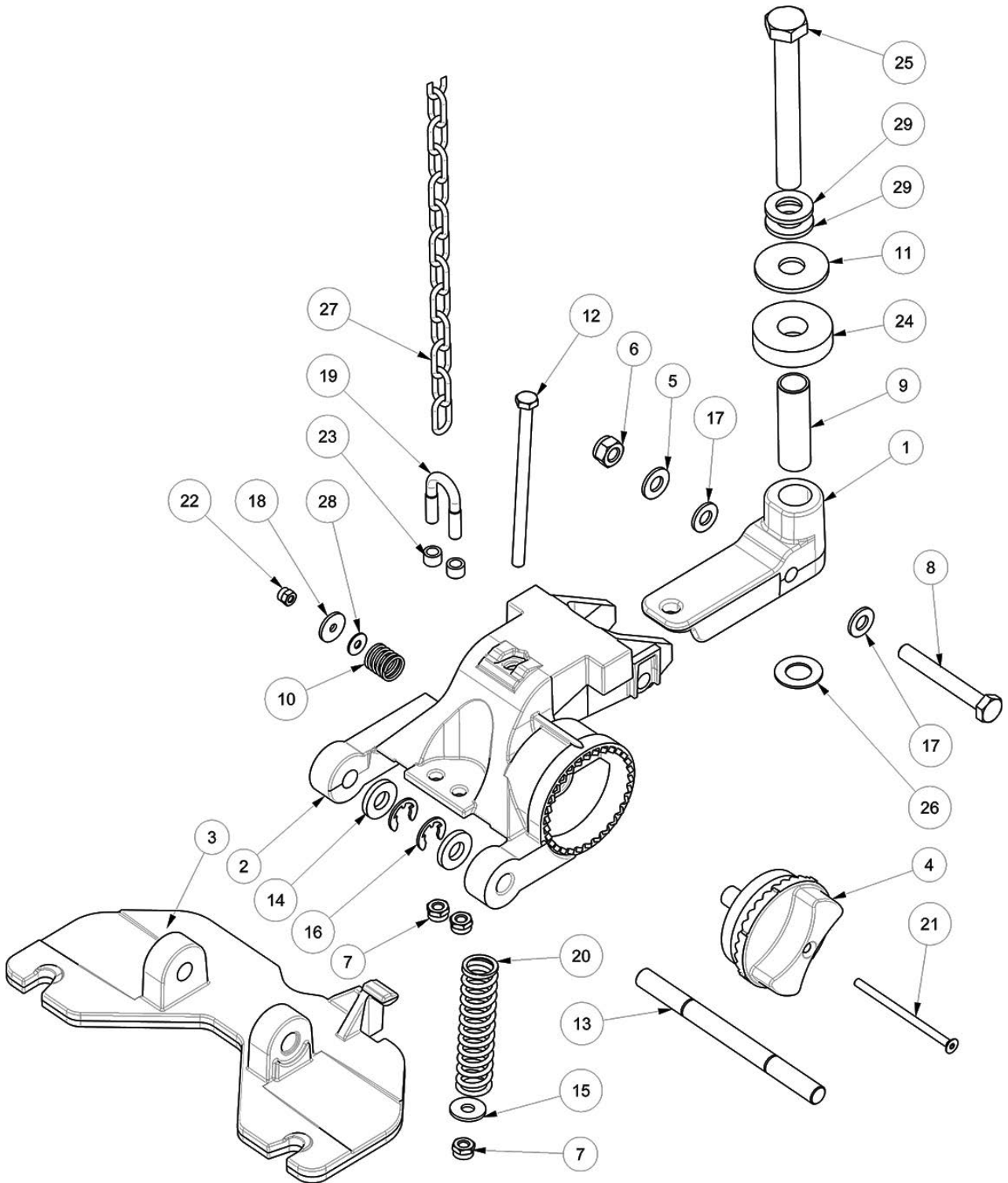
Abb. 38: Ersatzteilzeichnung 7
