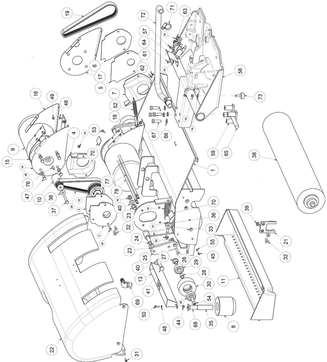
Abb. 33: Ersatzteilzeichnung 1 - Reinigungskopf
