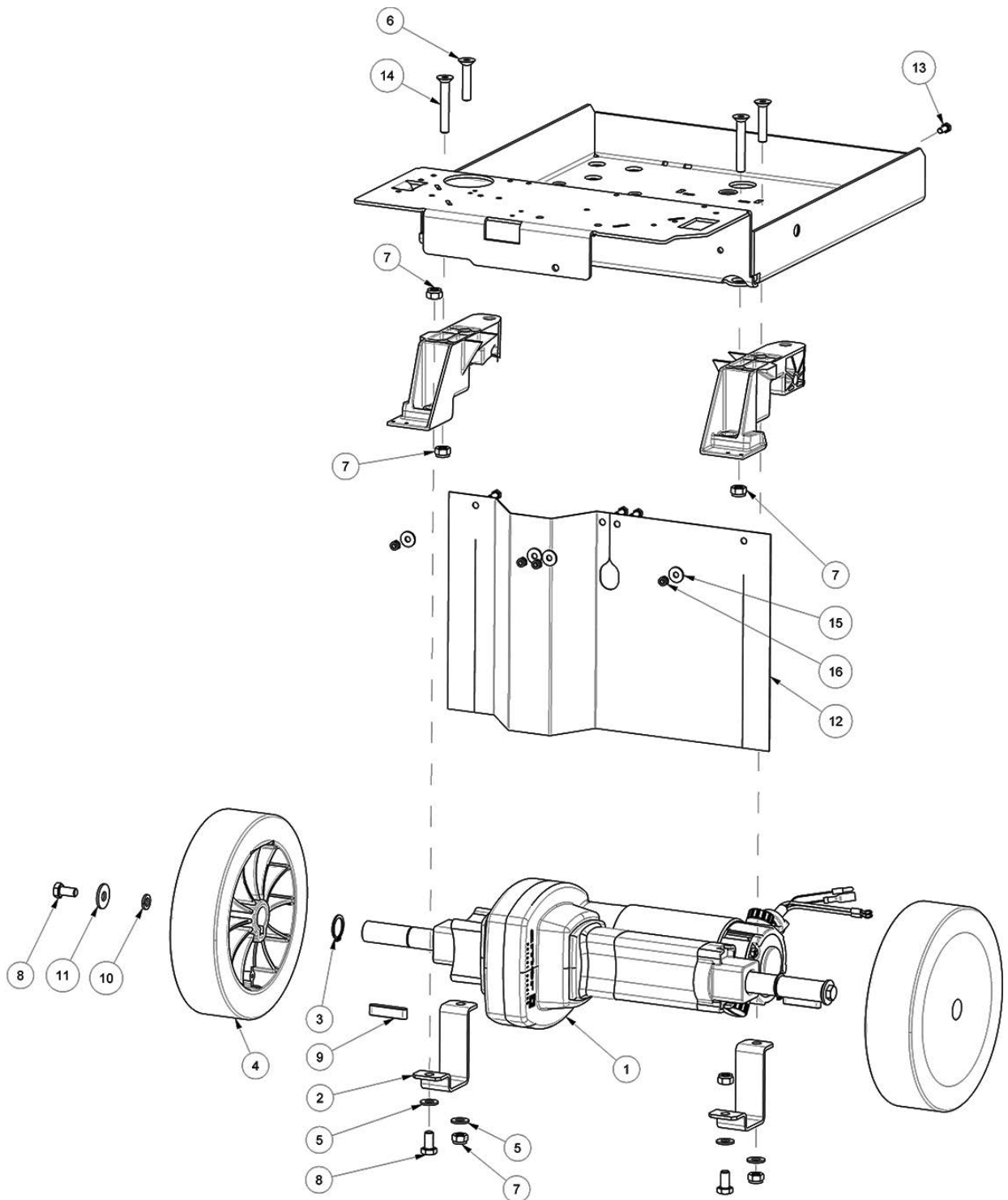
Abb. 37: Ersatzteilzeichnung 6
