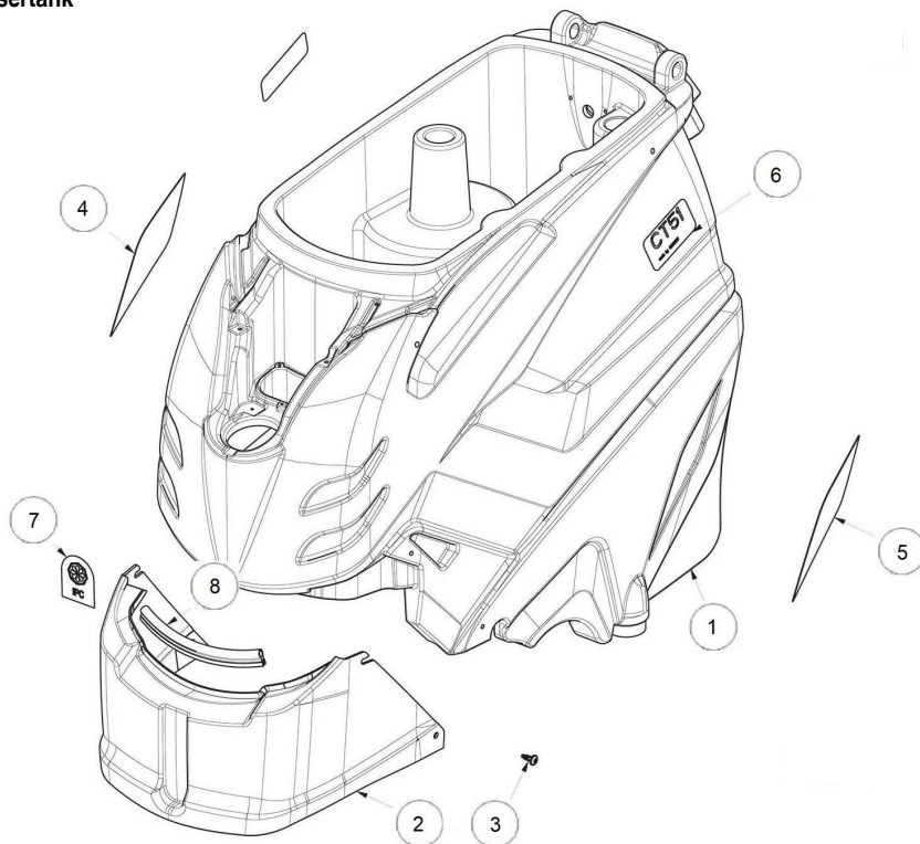
Abb. 54: Ersatzteilzeichnung 11 und Ersatzteilzeichnung 12
