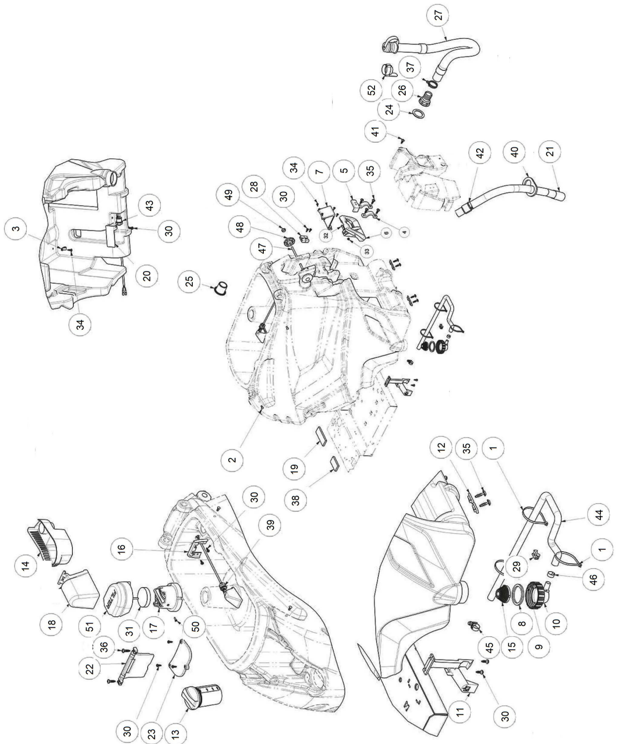
Abb. 39: Ersatzteilzeichnung 8
