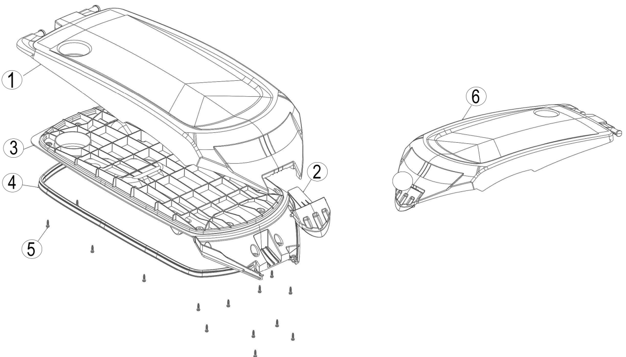
Abb. 49: Ersatzteilzeichnung 4 und Ersatzteilzeichnung 5
