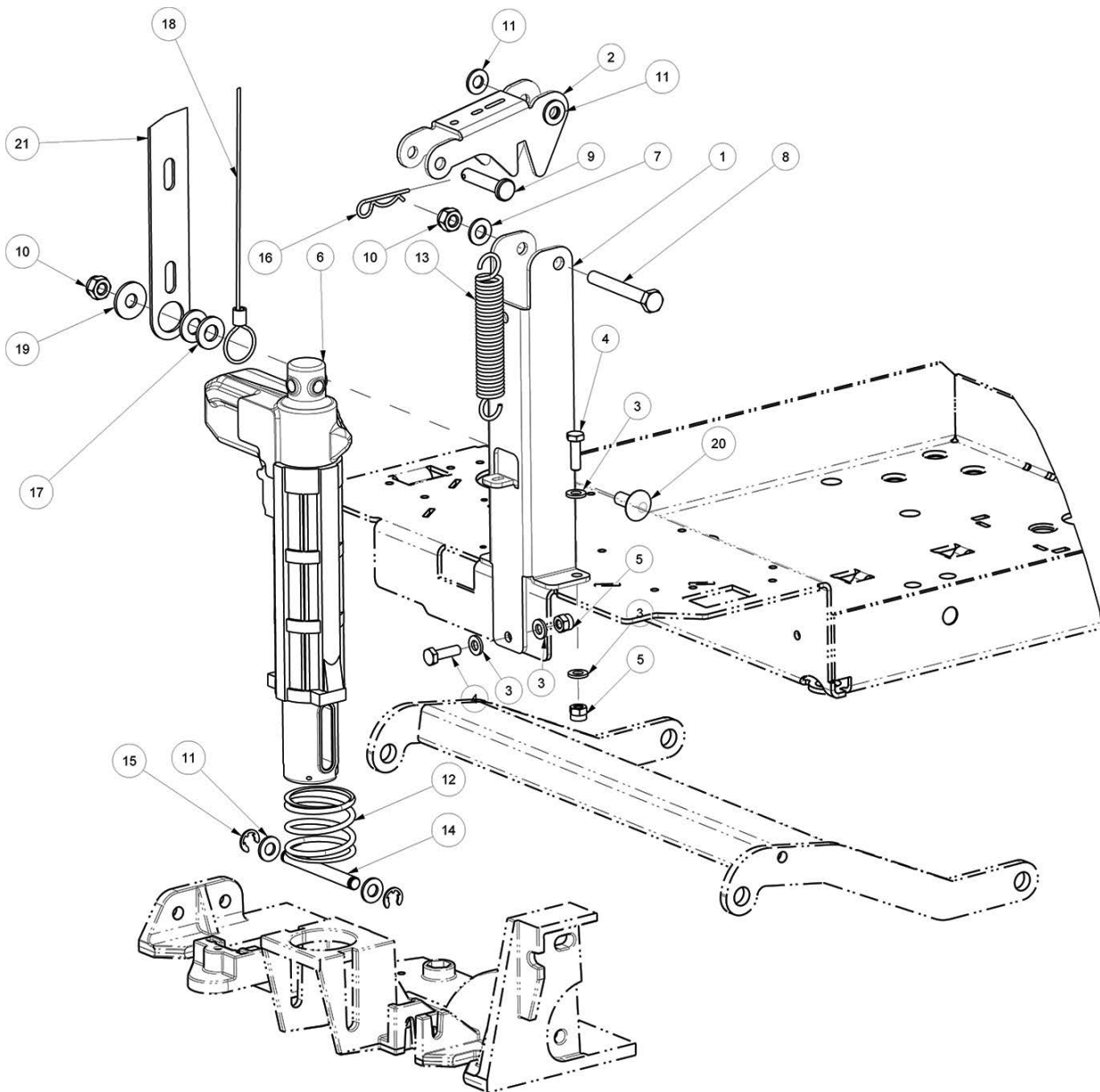
Abb. 36: Ersatzteilzeichnung 5
