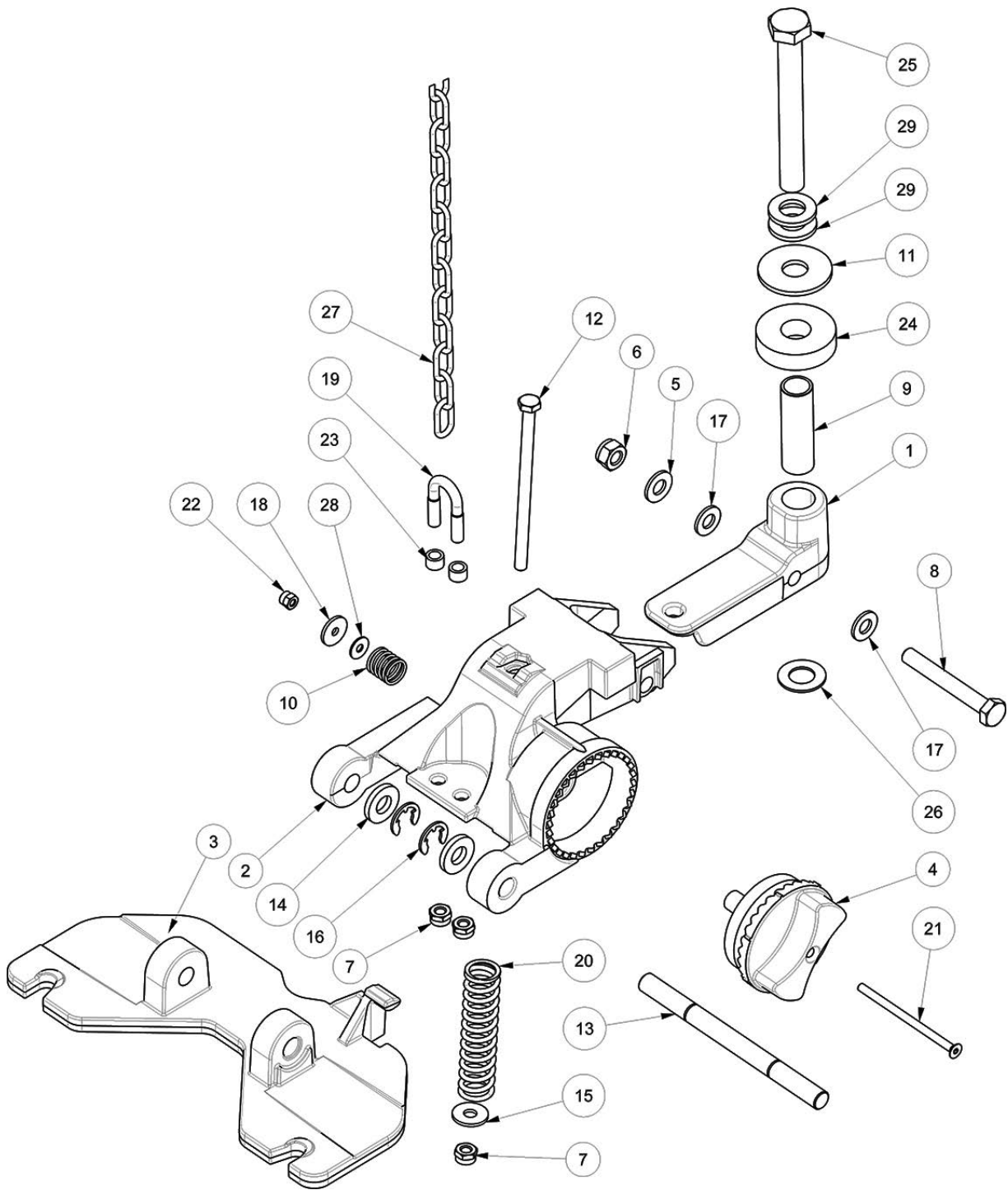
Abb. 47: Ersatzteilzeichnung 2
