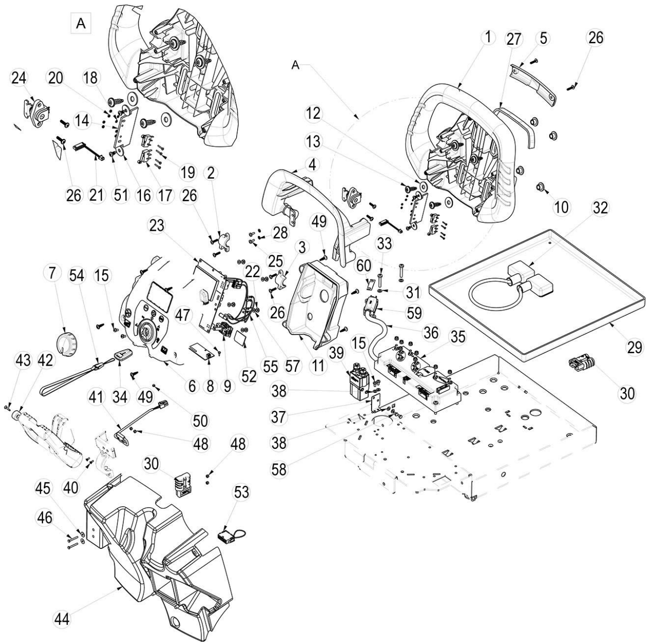
Abb. 43: Ersatzteilzeichnung 13
