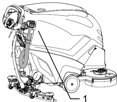
Abb. 13: Anschluss der Schläuche
