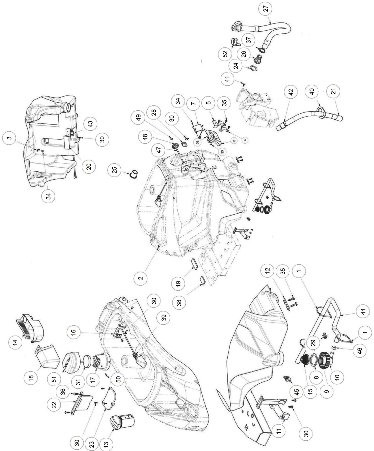
Abb. 53: Ersatzteilzeichnung 10
