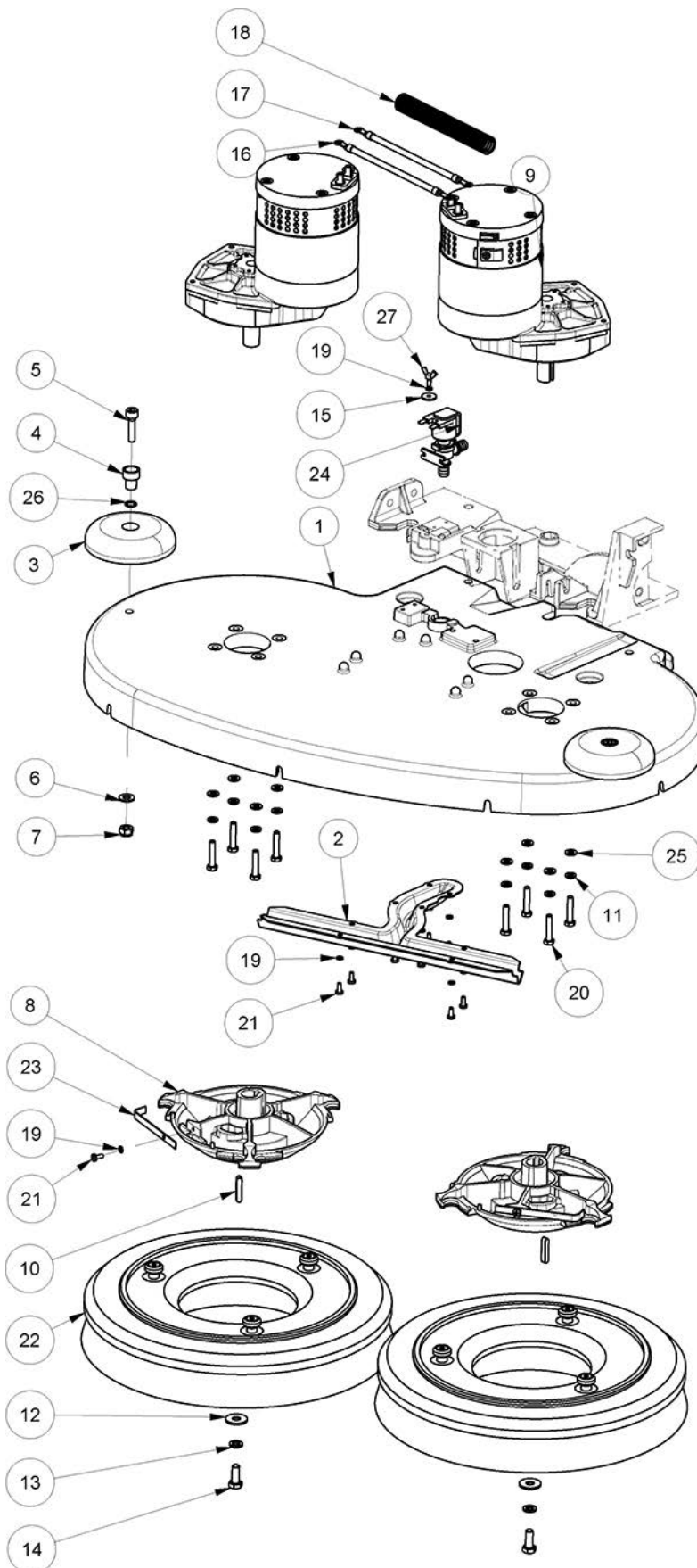
Abb. 51: Ersatzteilzeichnung 8
