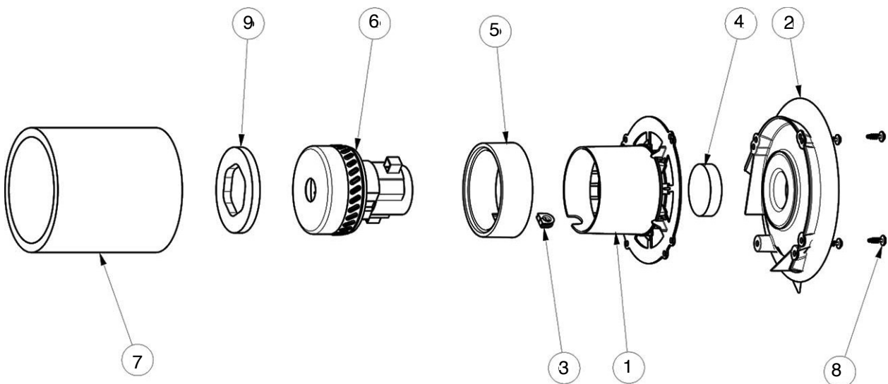
Abb. 50: Ersatzteilzeichnung 6 und Ersatzteilzeichnung 7
