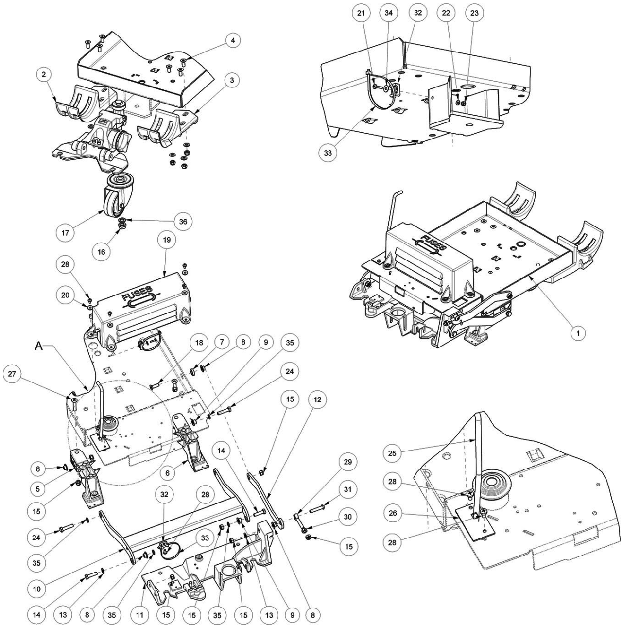
Abb. 34: Ersatzteilzeichnung 2: Gestell, Teil 1
