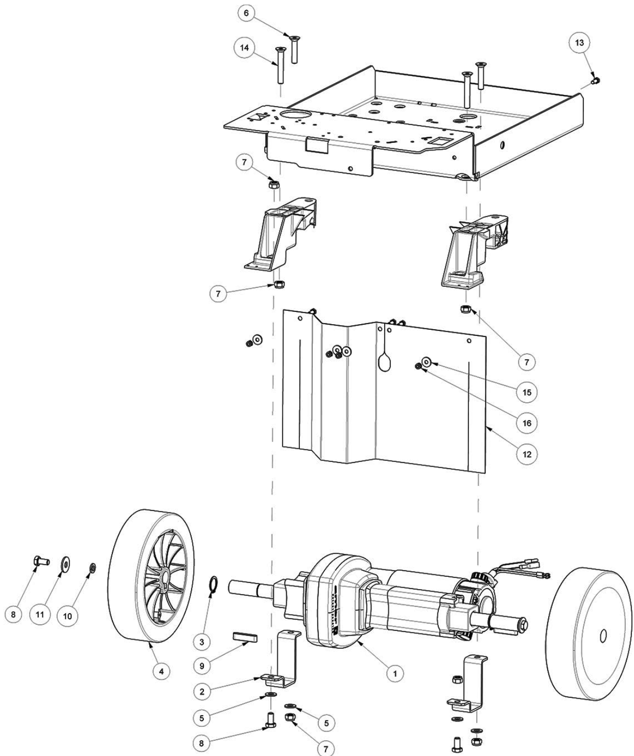
Abb. 24: Ersatzteilzeichnung 3
