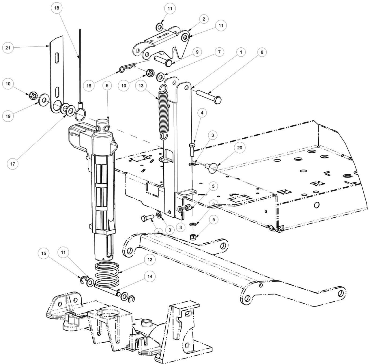
Abb. 23: Ersatzteilzeichnung 2: Gestell, Teil 1
