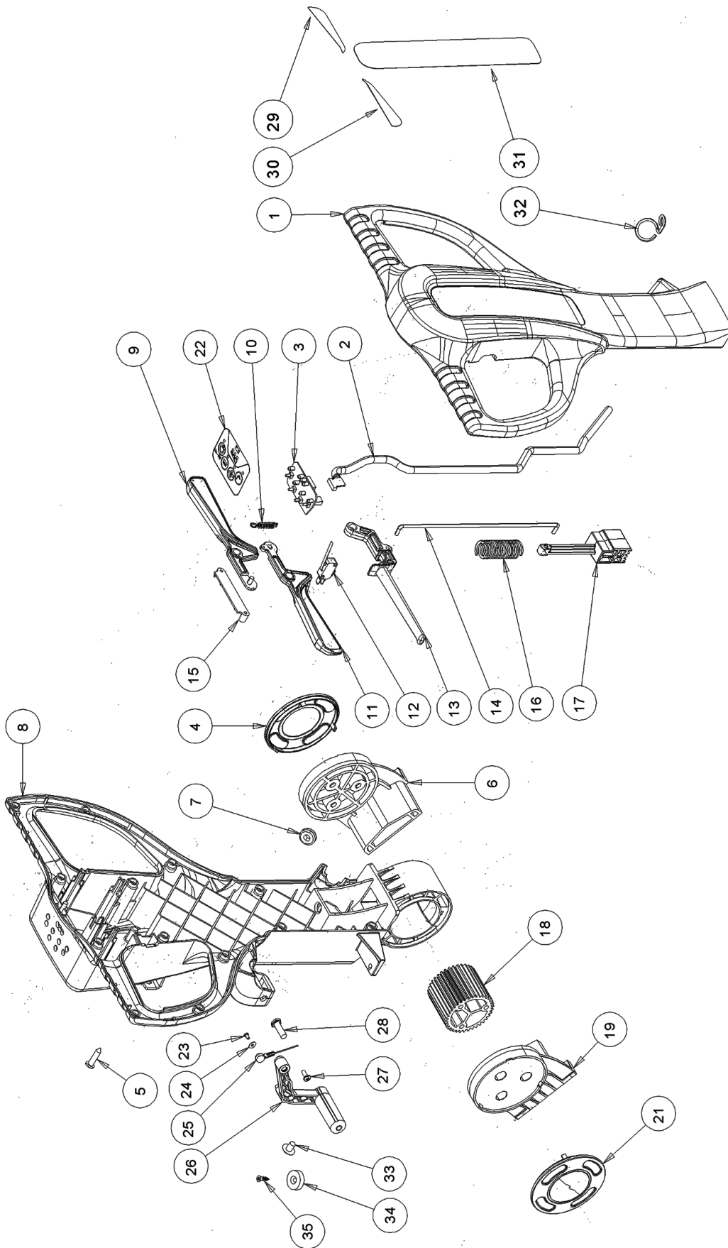
Abb. 45: Ersatzteilzeichnung 7
