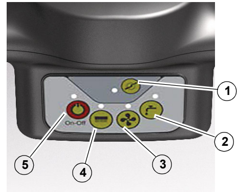
Abb. 6: Bedienfeld kabelgebundene Modelle
