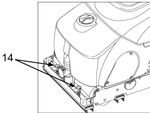
Abb. 14: Druckregelung einstellen
