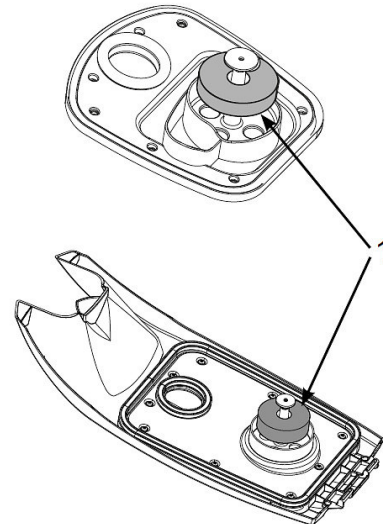
Abb. 35: Schwimmer reinigen
