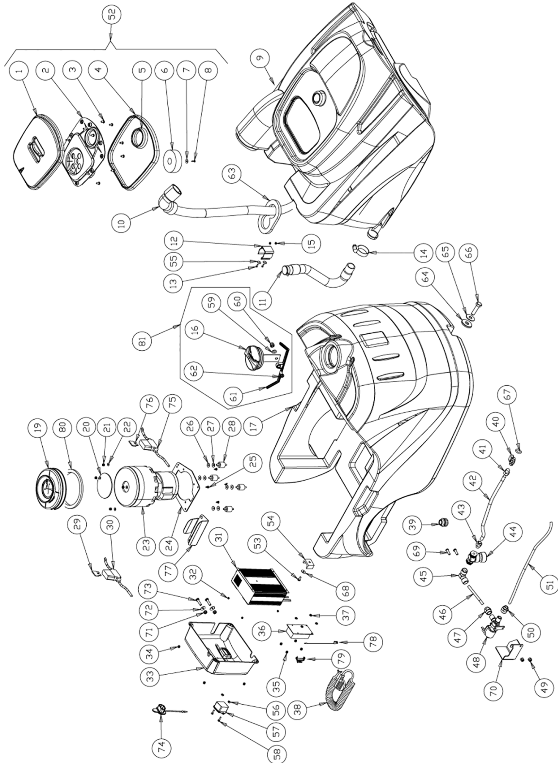
Abb. 39: Ersatzteilzeichnung 1
