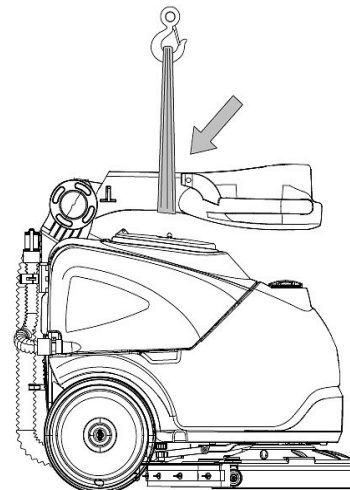
Abb. 8: Anheben der Maschine
