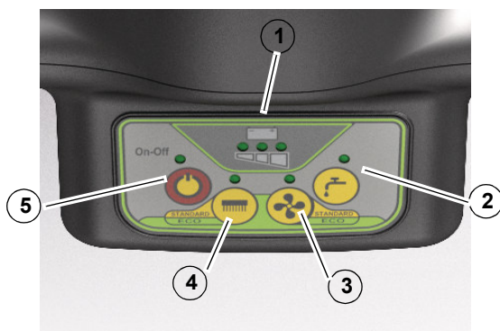
Abb. 5: Bedienfeld mit Batterieledestandanzeige
