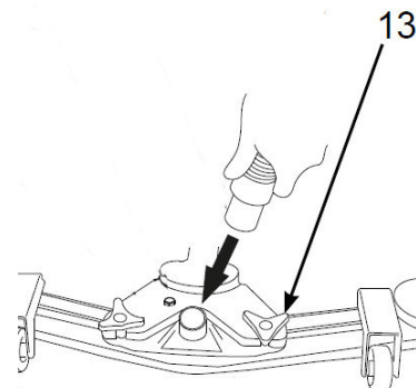
Abb. 12: Befestigen der Saugleiste
