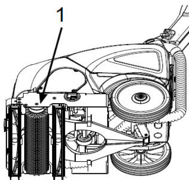
Abb. 20: Einbau der Bürstenwalze
