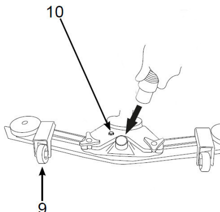
Abb. 15: Höhenverstellung der Saugleiste
