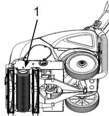
Abb. 21: Einbau der Bürstenwalze
