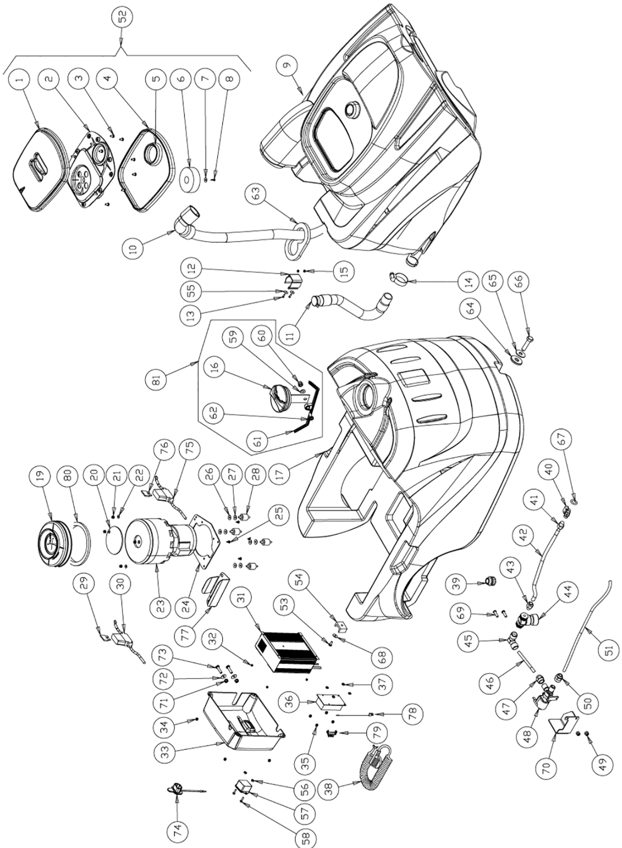
Abb. 40: Ersatzteilzeichnung 2
