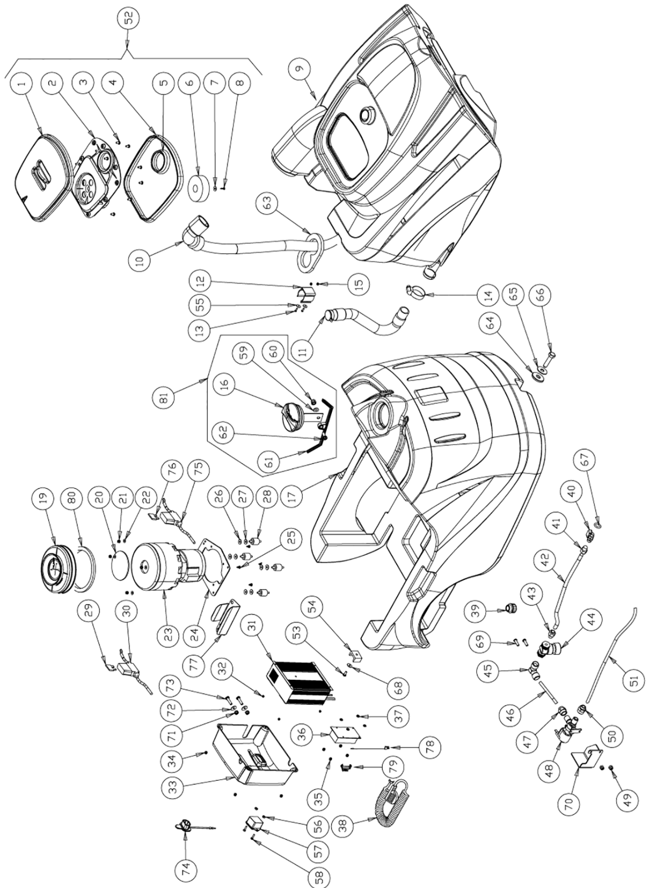
Abb. 41: Ersatzteilzeichnung 3
