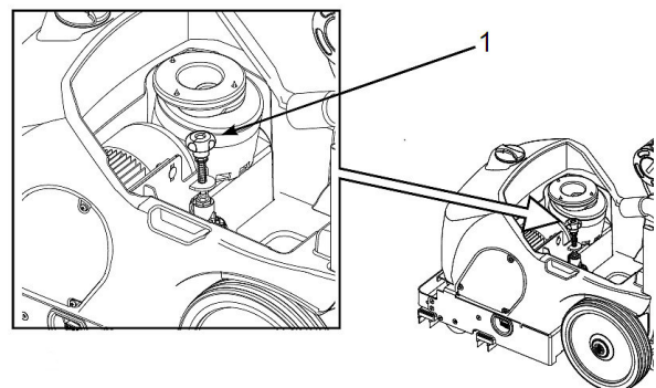
Abb. 22: Anpressdruck der Bürstenwalze einstellen
