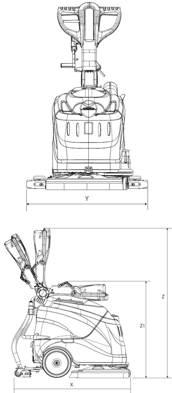
Abb. 3: Abmessungen SSM 500
