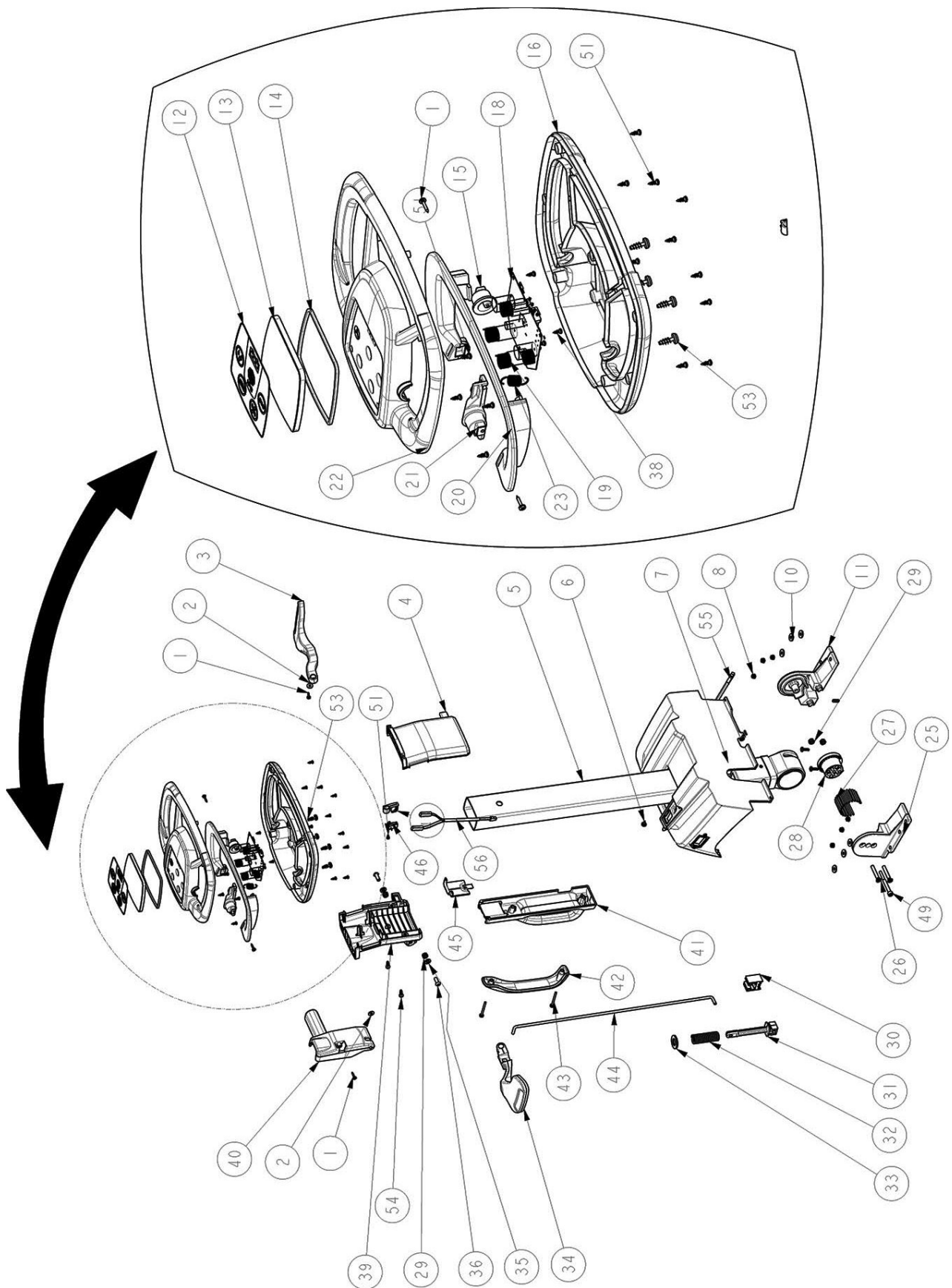
Abb. 33: Ersatzteilzeichnung 2: Handgriff
