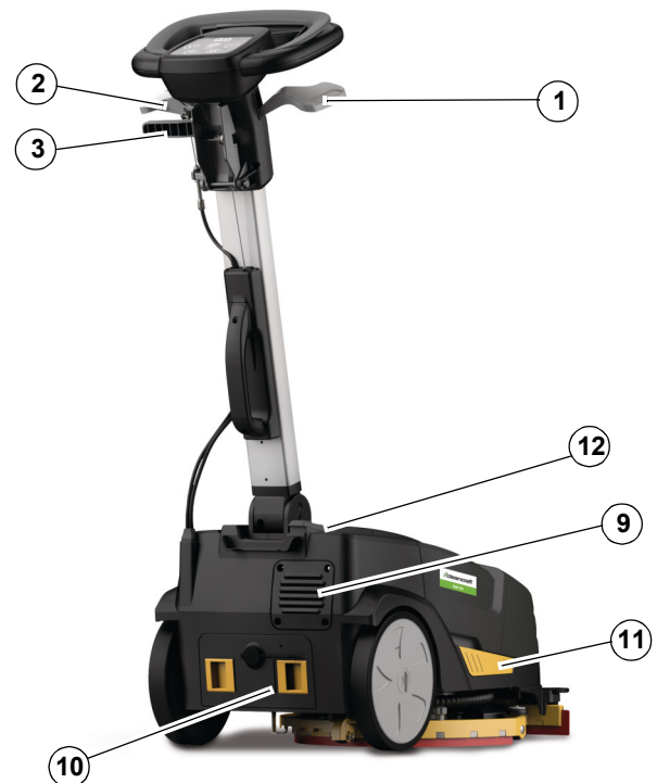
Abb. 5: Hinteransicht der Maschine
