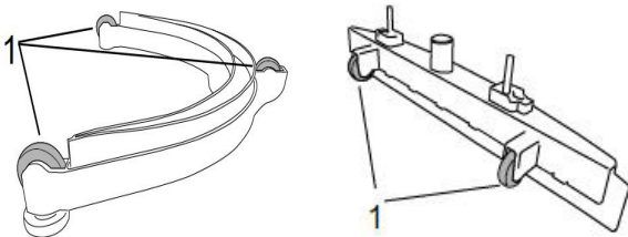
Abb. 25: Saugleiste einstellen
