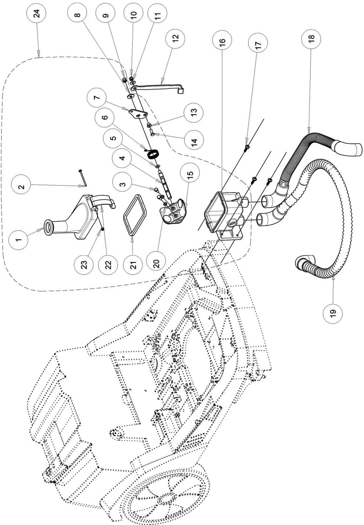
Abb. 35: Ersatzteilzeichnung 4: Reinigungseinheit
