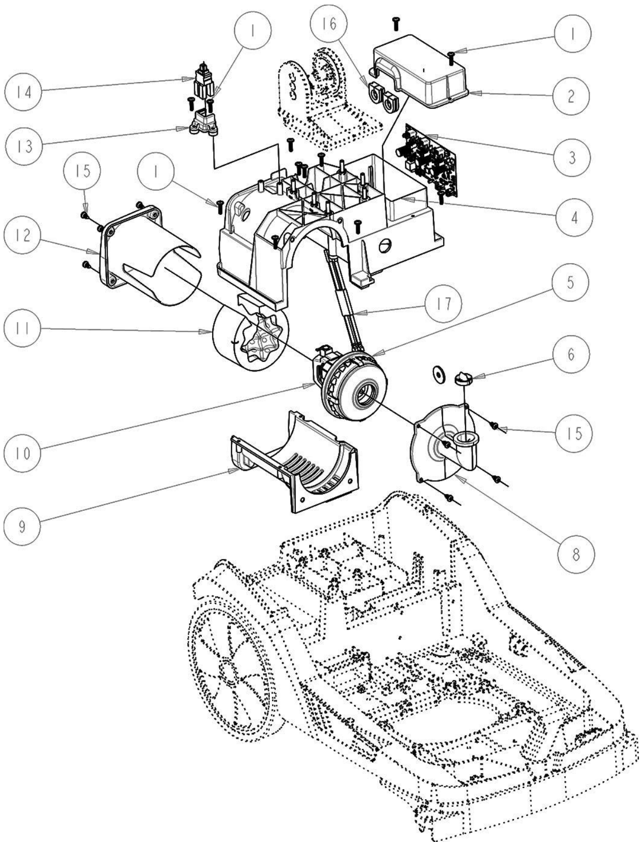
Abb. 37: Ersatzteilzeichnung 6: Saugmotor
