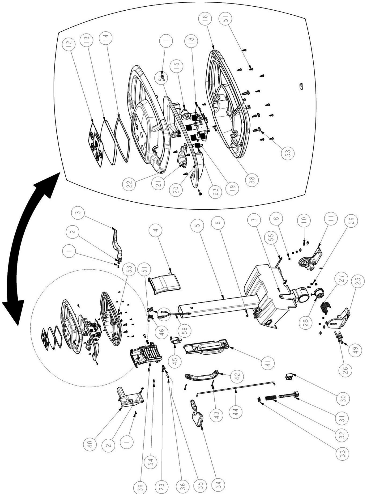
Abb. 34: Ersatzteilzeichnung 3: Handgriff
