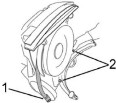
Abb. 29: Bauteile lösen
