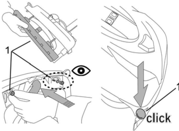
Abb. 8: Zusammenbau
