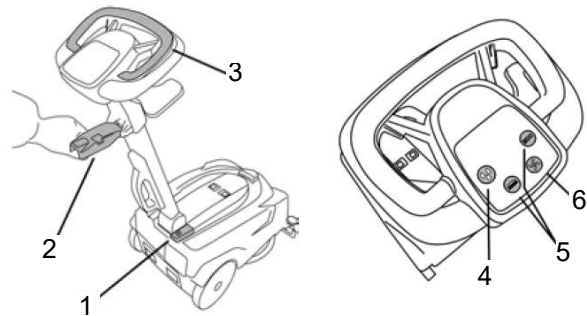
Abb. 16: Arbeiten mit der Maschine
