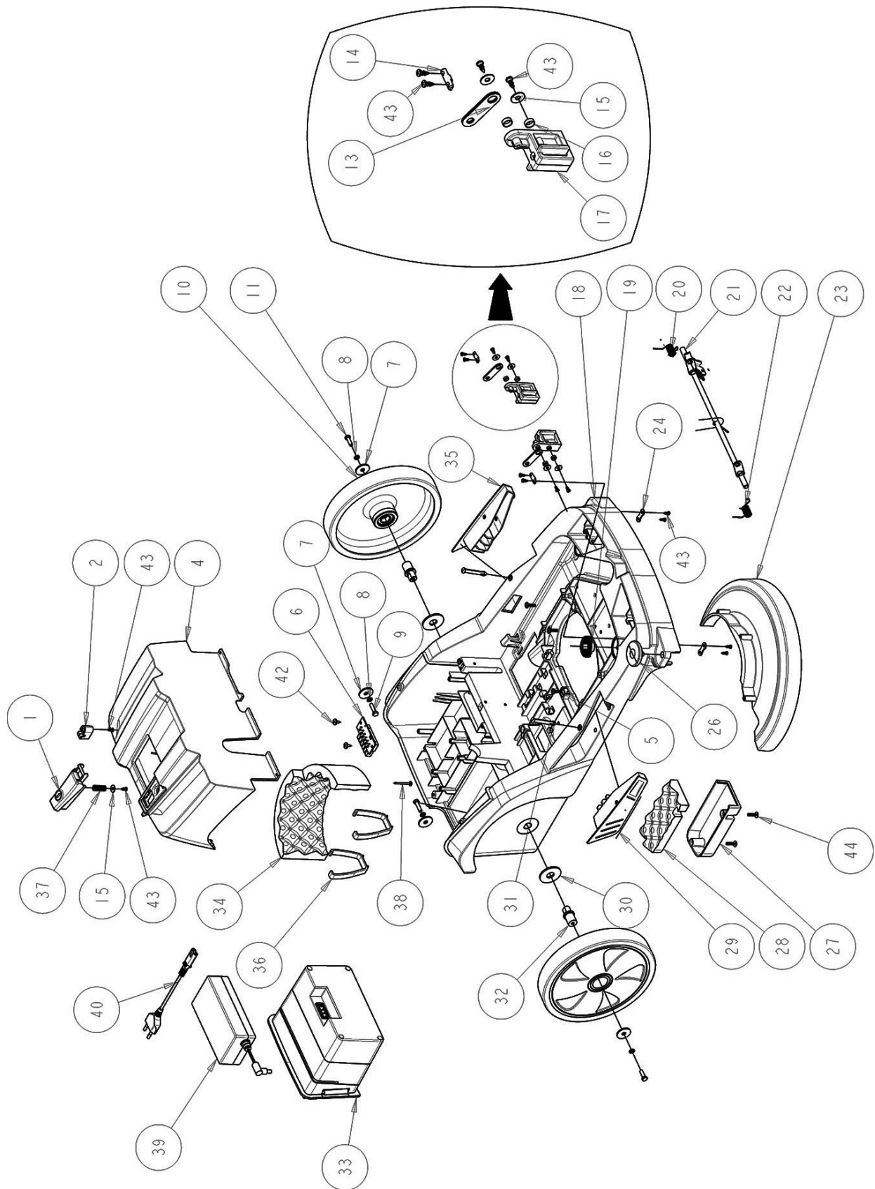
Abb. 32: Ersatzteilzeichnung 1: Fahrwerk
