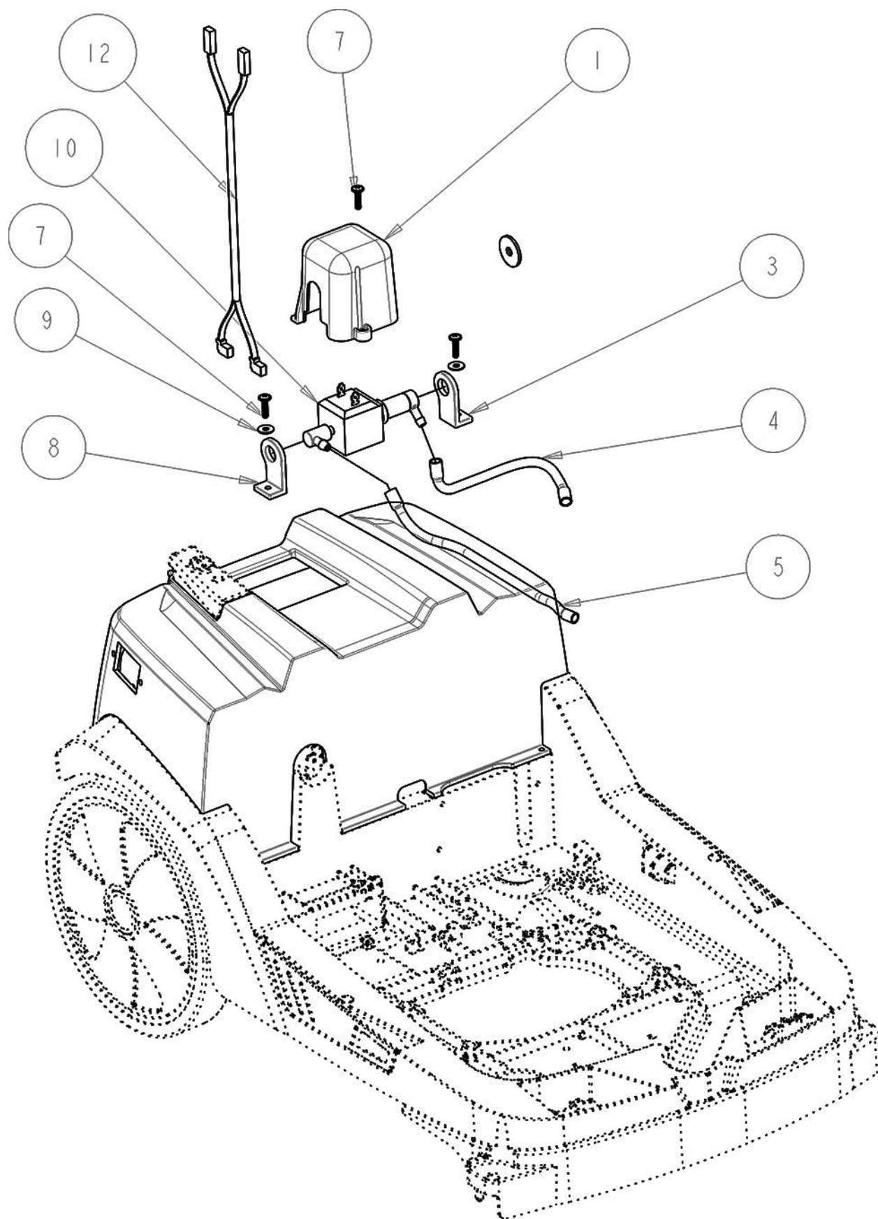
Abb. 40: Ersatzteilzeichnung 9: Pumpe
