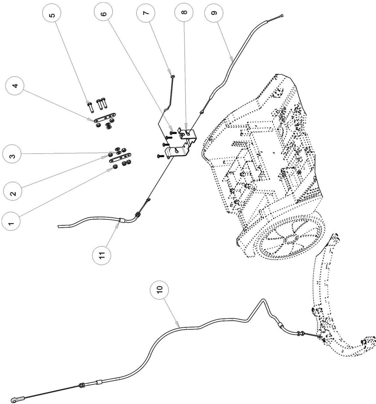
Abb. 41: Ersatzteilzeichnung 10: Kabel
