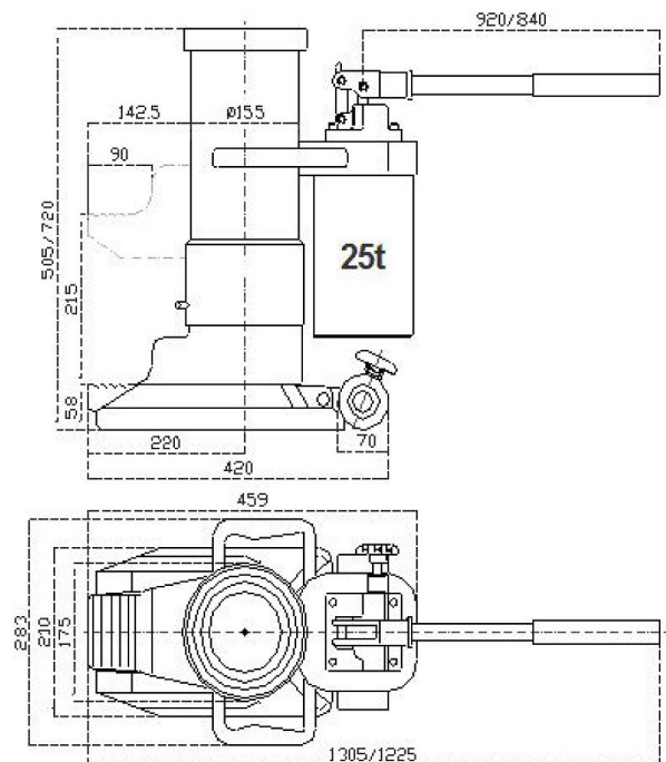
Abb. 5: Abmessungen HMH 25
