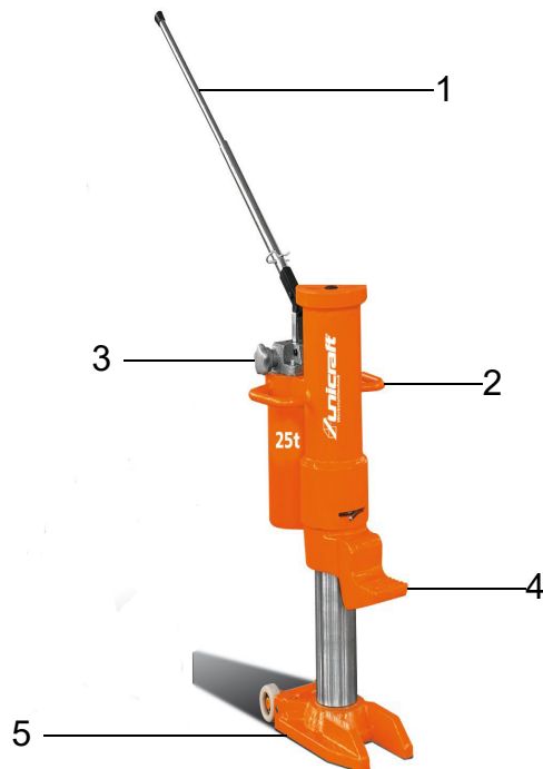
Abb. 2: Gerätebeschreibung
