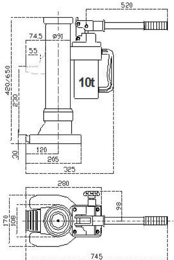
Abb. 4: Abmessungen HMH 10
