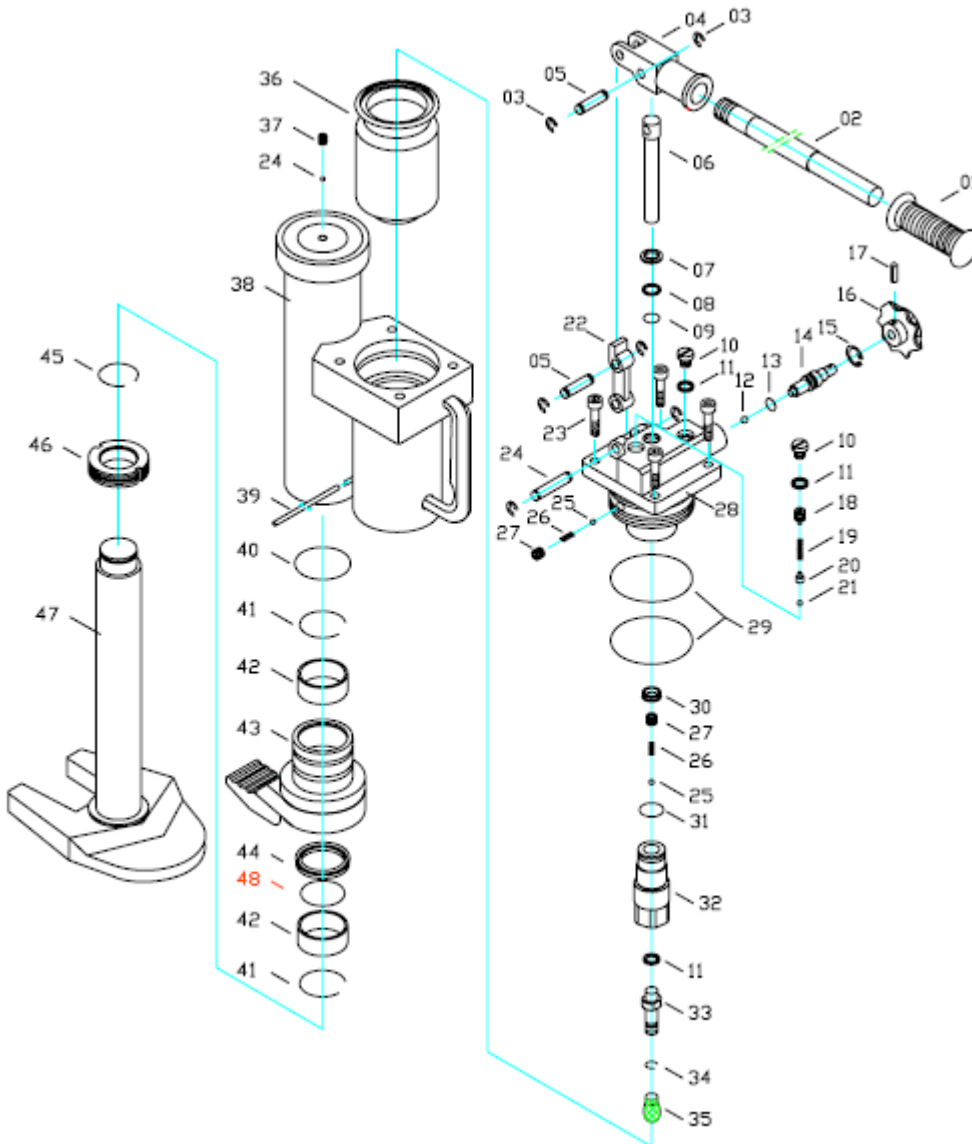
Abb. 7: Ersatzteilzeichnung HMH 5/10
