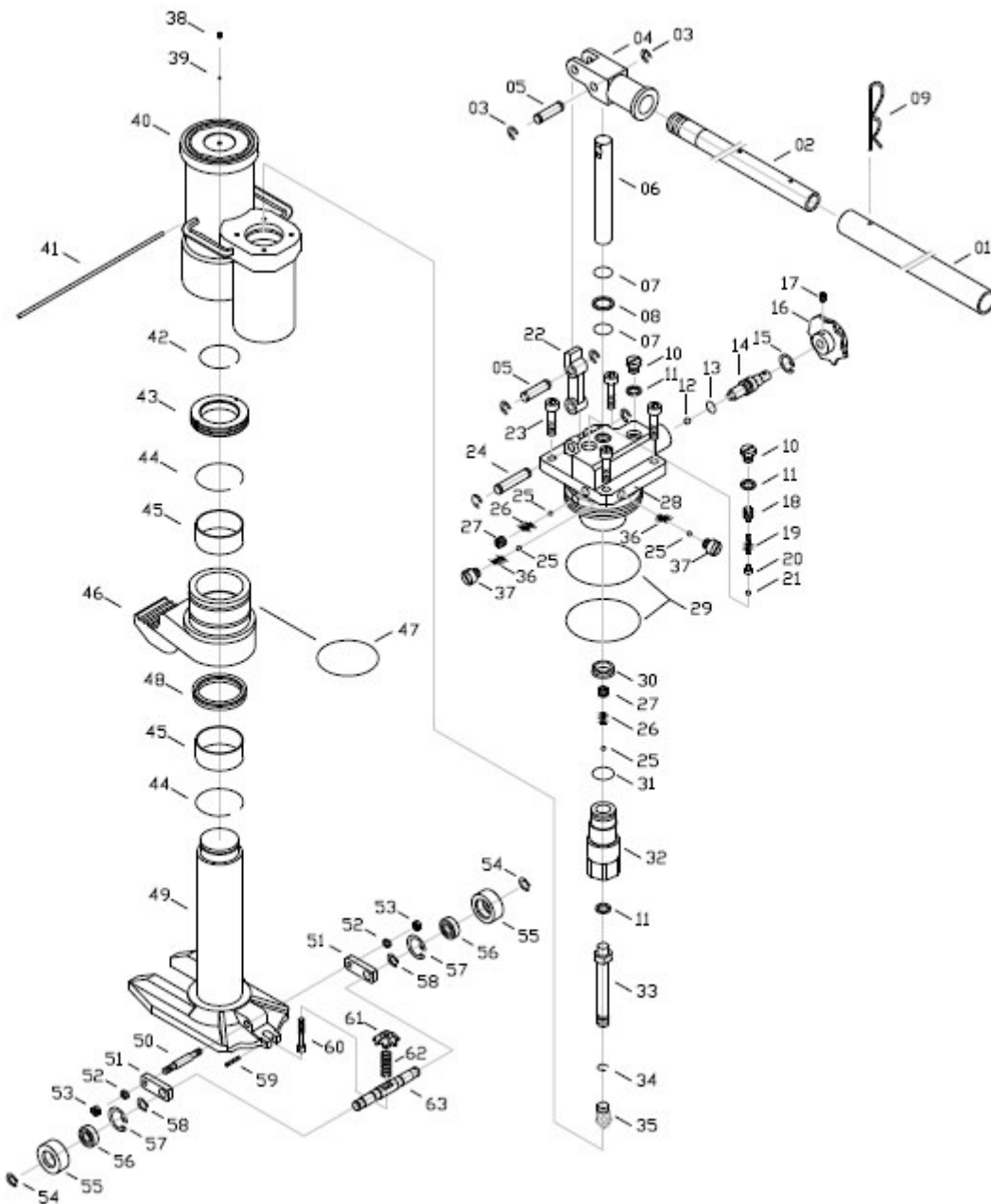
Abb. 8: HMH 25
