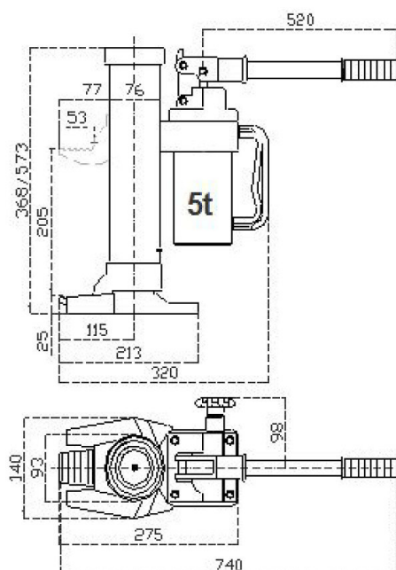
Abb. 3: Abmessungen HMH 5
