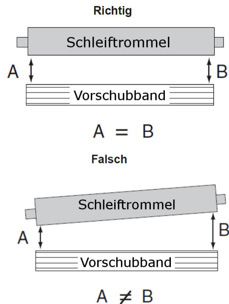
Abb. 24: Parallelität von Vorschubband und Schleiftrommel
