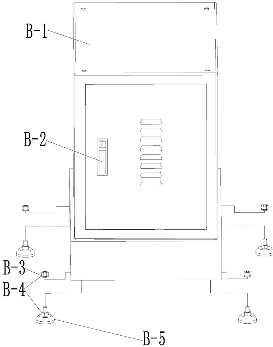
Abb. 35: Ersatzteilzeichnung 2
