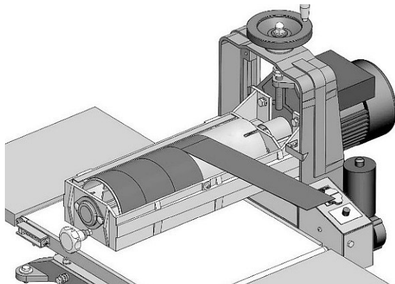
Abb. 17: Schleifpapier aufwickeln
