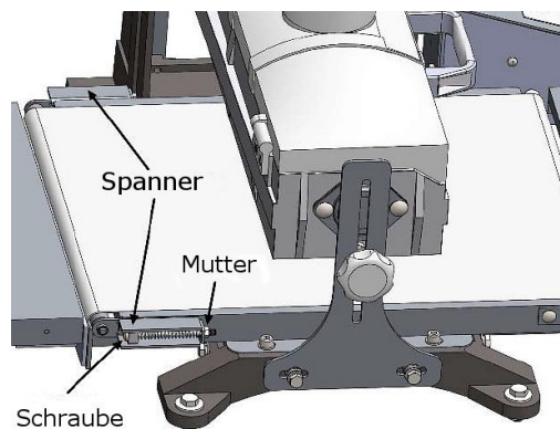
Abb. 29: Vorschubband spannen
