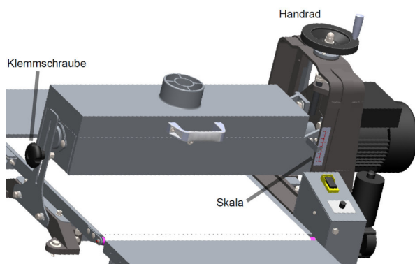
Abb. 13: Höhenverstellung
