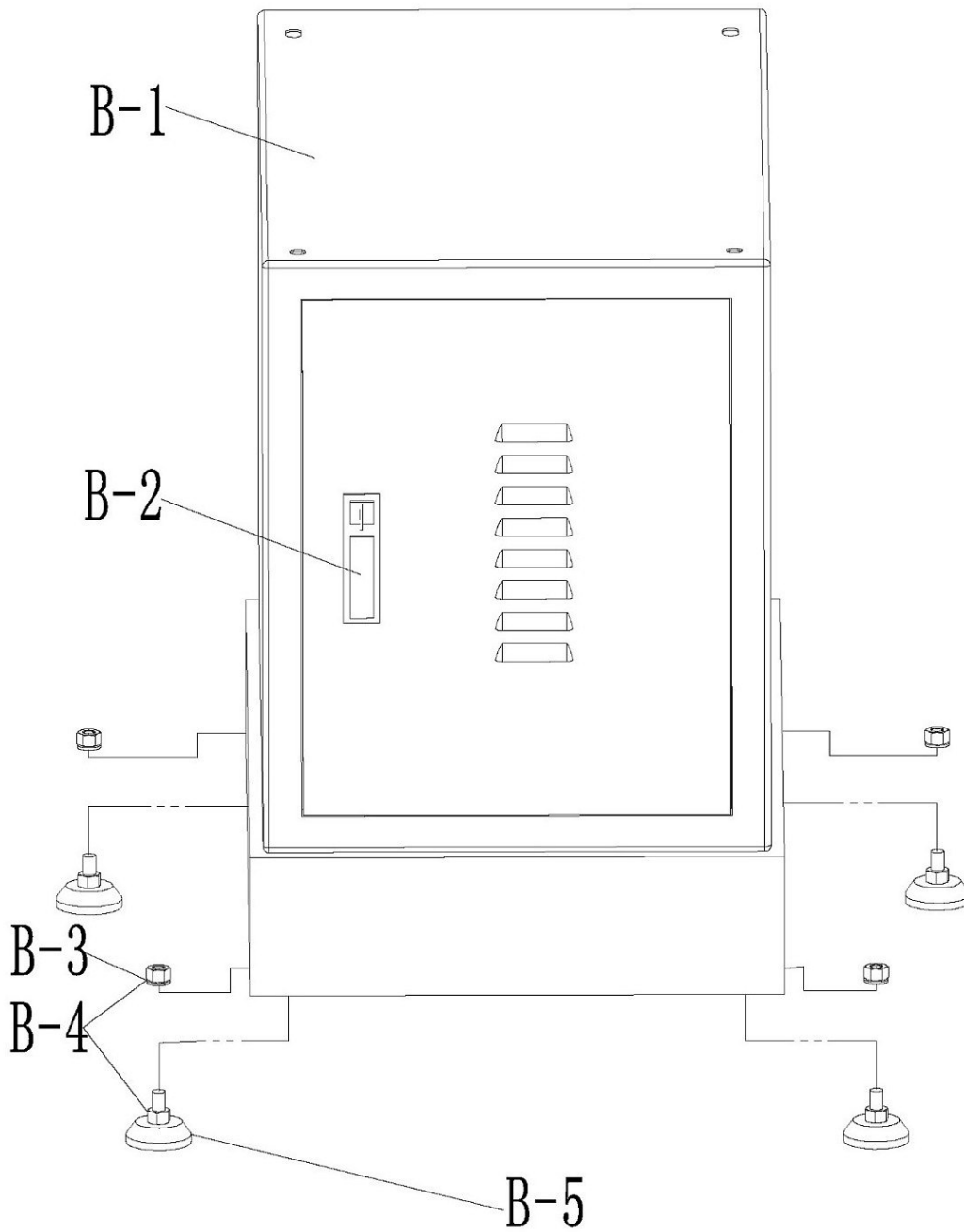
Abb. 37: Ersatzteilzeichnung 2
