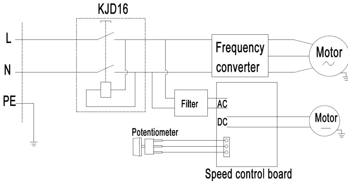
Abb. 39: Elektroschaltplan ZSM 560 VARIO
