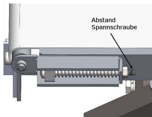
Abb. 30: Position der Spannschrauben
