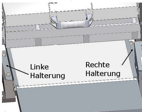
Abb. 25: Parallelität Vorschubband zu Schleiftrommel einstellen
