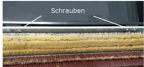
Abb. 33: Schleifwalze einsetzen
