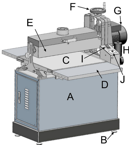
Abb. 3: Zylinderschleifmaschine ZSM 560
