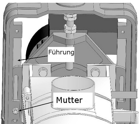
Abb. 22: Führungsseiten lösen
