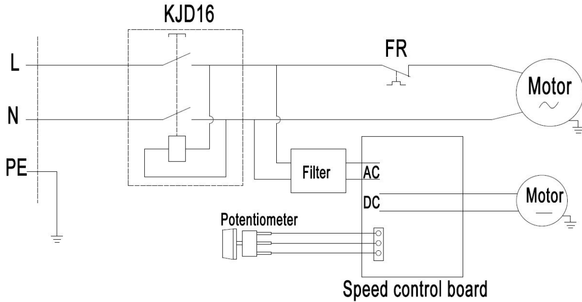
Abb. 38: Elektroschaltplan ZSM 560
