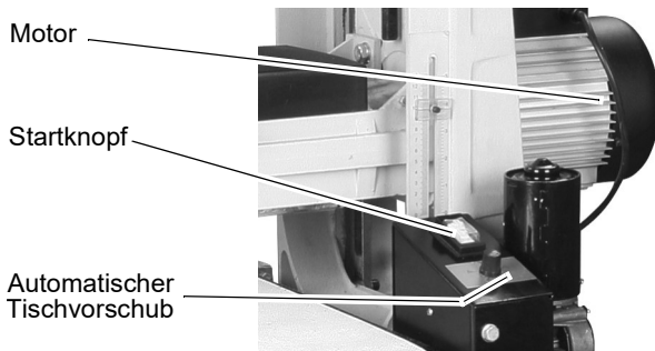
Abb. 9: Starten der Maschine ZSM 560
