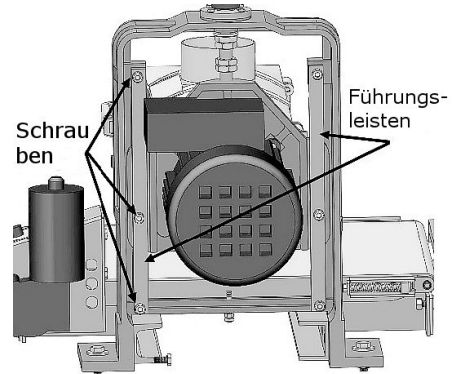
Abb. 23: Führungsseiten einstellen
