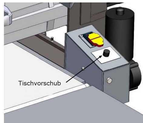
Abb. 18: Vorschubgeschwindigkeit einstellen
