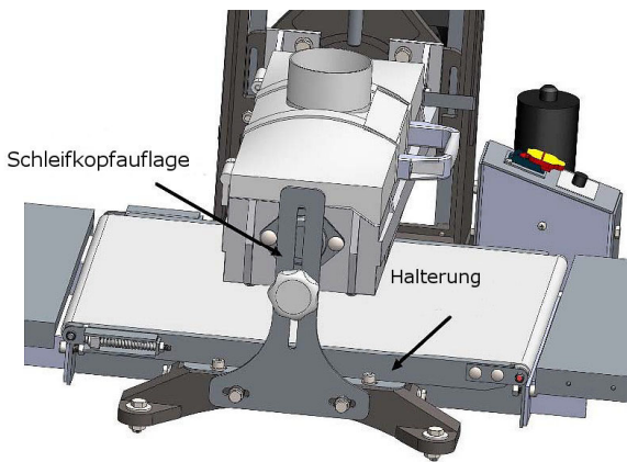
Abb. 40: Vorschubband austauschen
