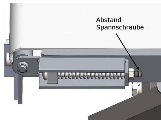
Abb. 43: Position der Spannschrauben
