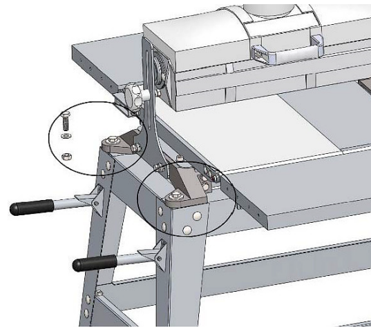
Abb. 13: Maschine auf Untergestell montieren
