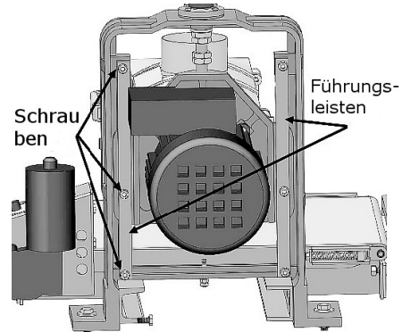
Abb. 36: Führungsseiten einstellen
