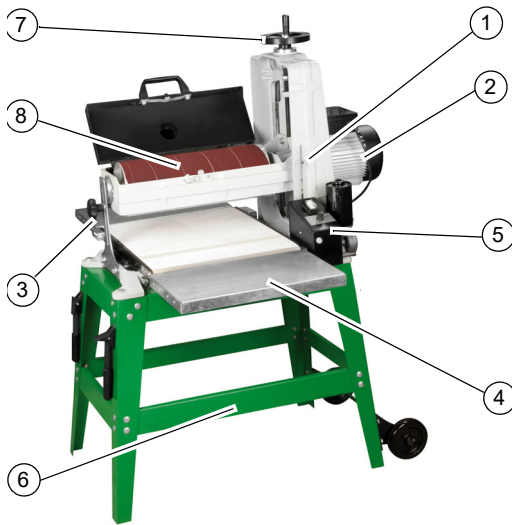
Abb. 5: Zylinderschleifmaschine ZSM 405
