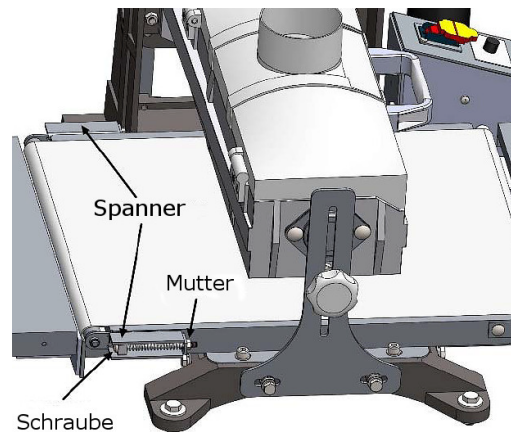
Abb. 42: Vorschubband spannen
