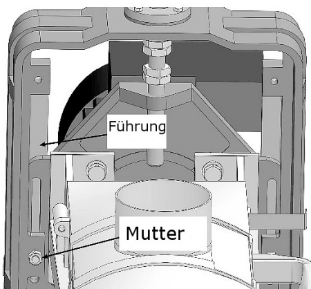
Abb. 35: Führungsseiten lösen
