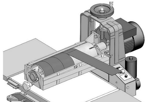
Abb. 23: Schleifpapier aufwickeln
