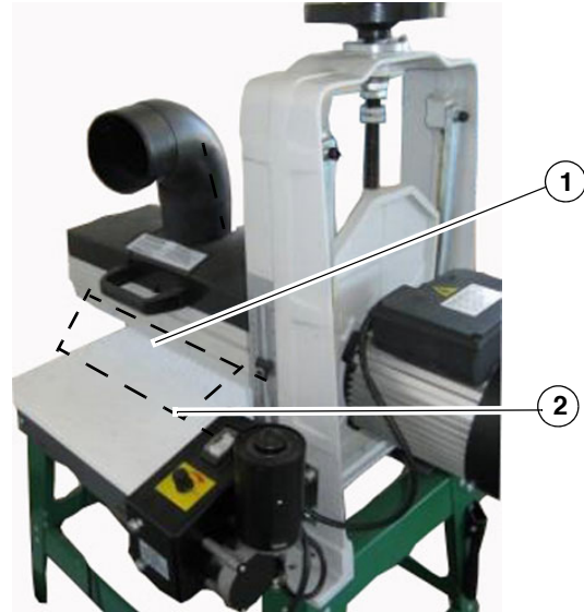
Abb. 2: Gefahrenbereiche
