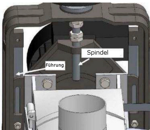
Abb. 39: Schmierung
