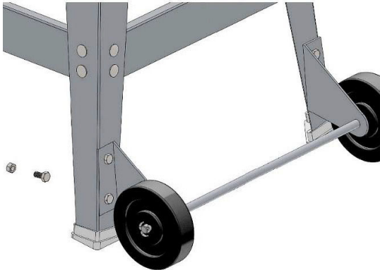
Abb. 11: Transporträder der Maschine montieren
