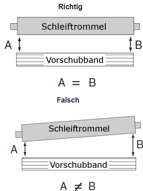
Abb. 37: Parallelität von Vorschubband und Schleiftrommel
