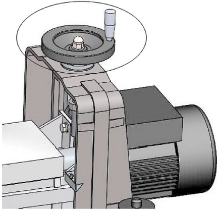
Abb. 15: Handrad montieren
