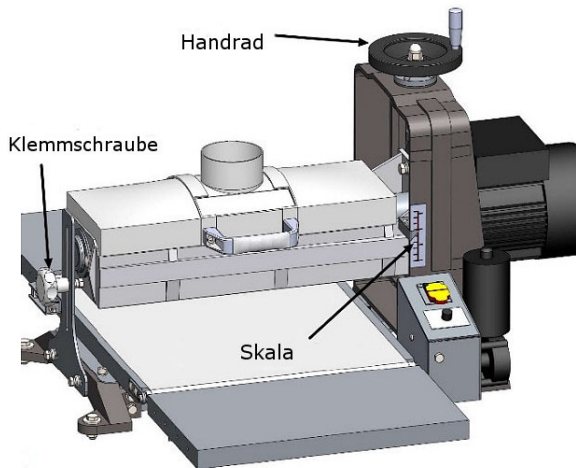
Abb. 19: Höhenverstellung
