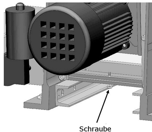
Abb. 34: Einstellschraube Höhenanschlag
