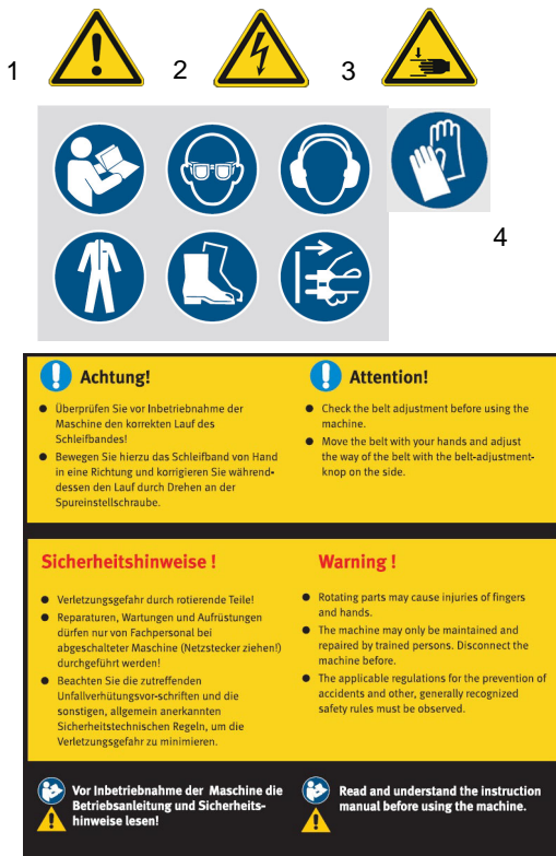
Abb. 1: Sicherheitskennzeichnungen 1 Warnung vor Gefahren | 2 Warnung vor gefährlicher elektrischer Spannung | 3 Warnung vor Quetschgefahr für die oberen Gliedmaßen | 4 Gebotszeichen / Sicherheitshinweise
