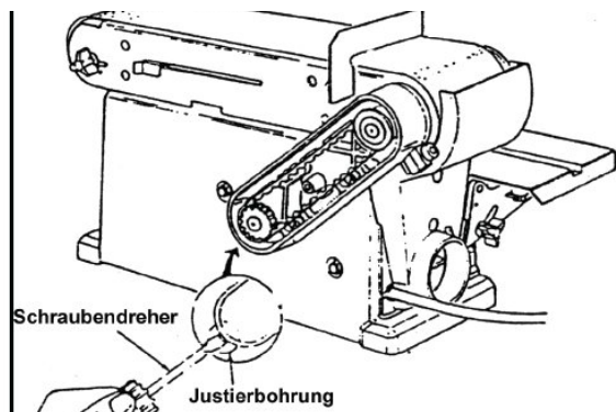
Abb. 20: Riemenwechsel
