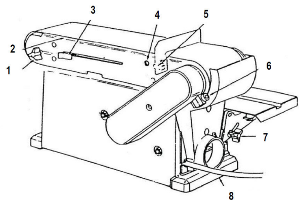
Abb. 3: Bedienelemente
