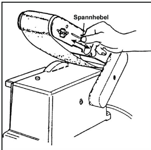
Abb. 12: Schleifbandwechsel
