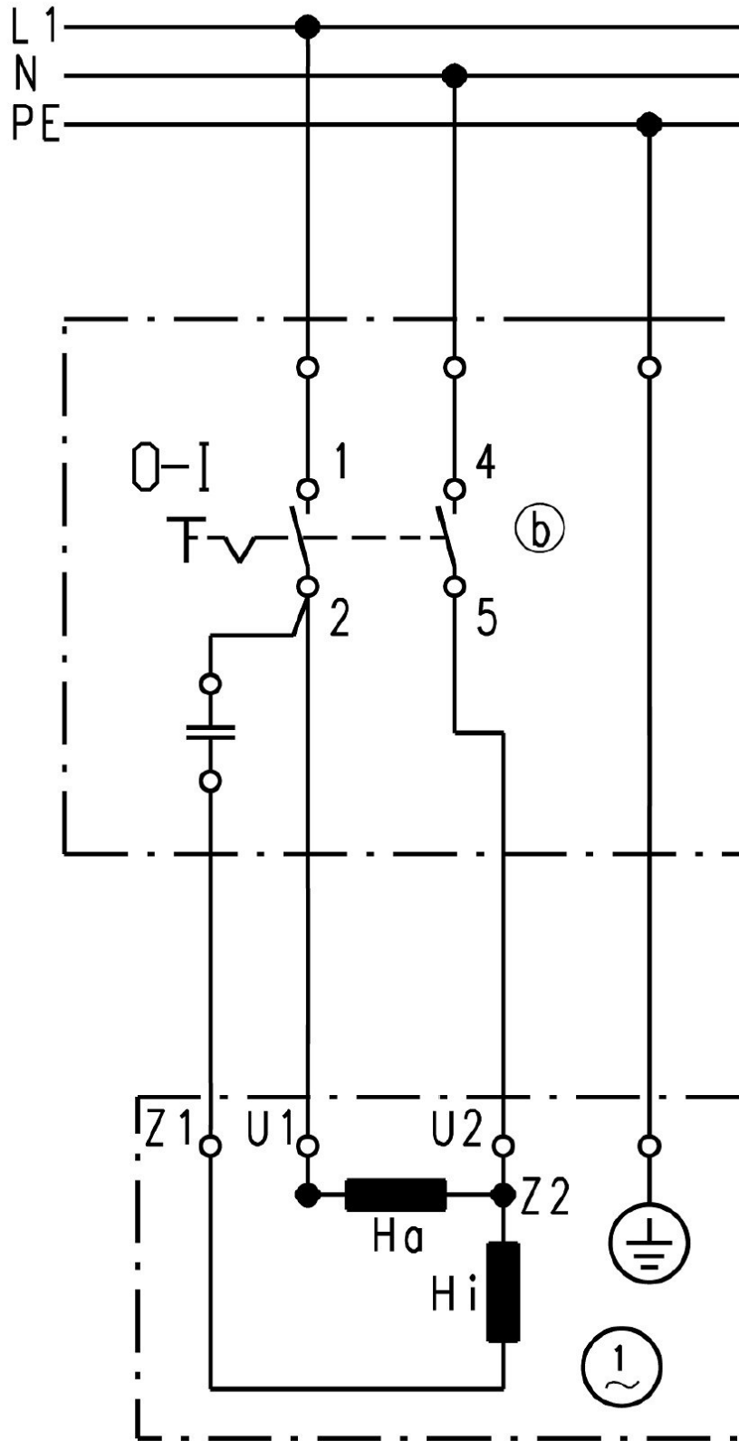
Abb. 16: Elektroschaltplan ASA 141
