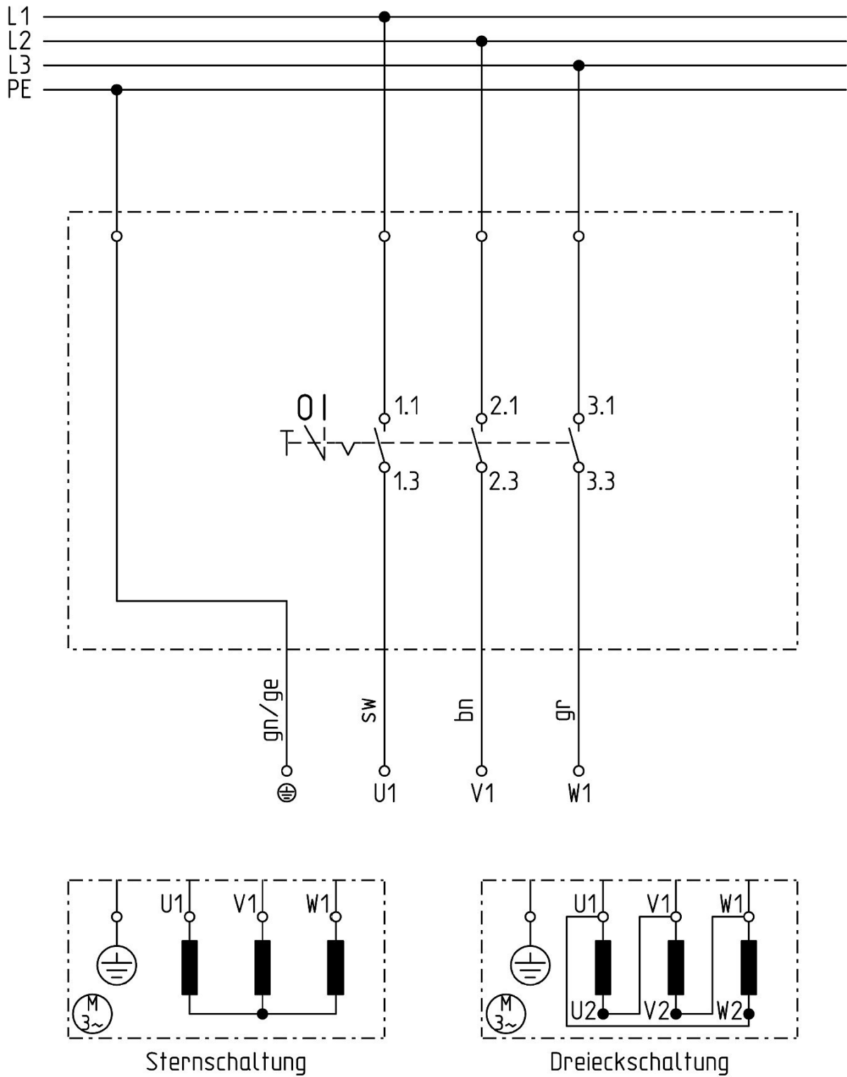
Abb. 17: Elektroschaltplan ASA 143 - 163 - 203
