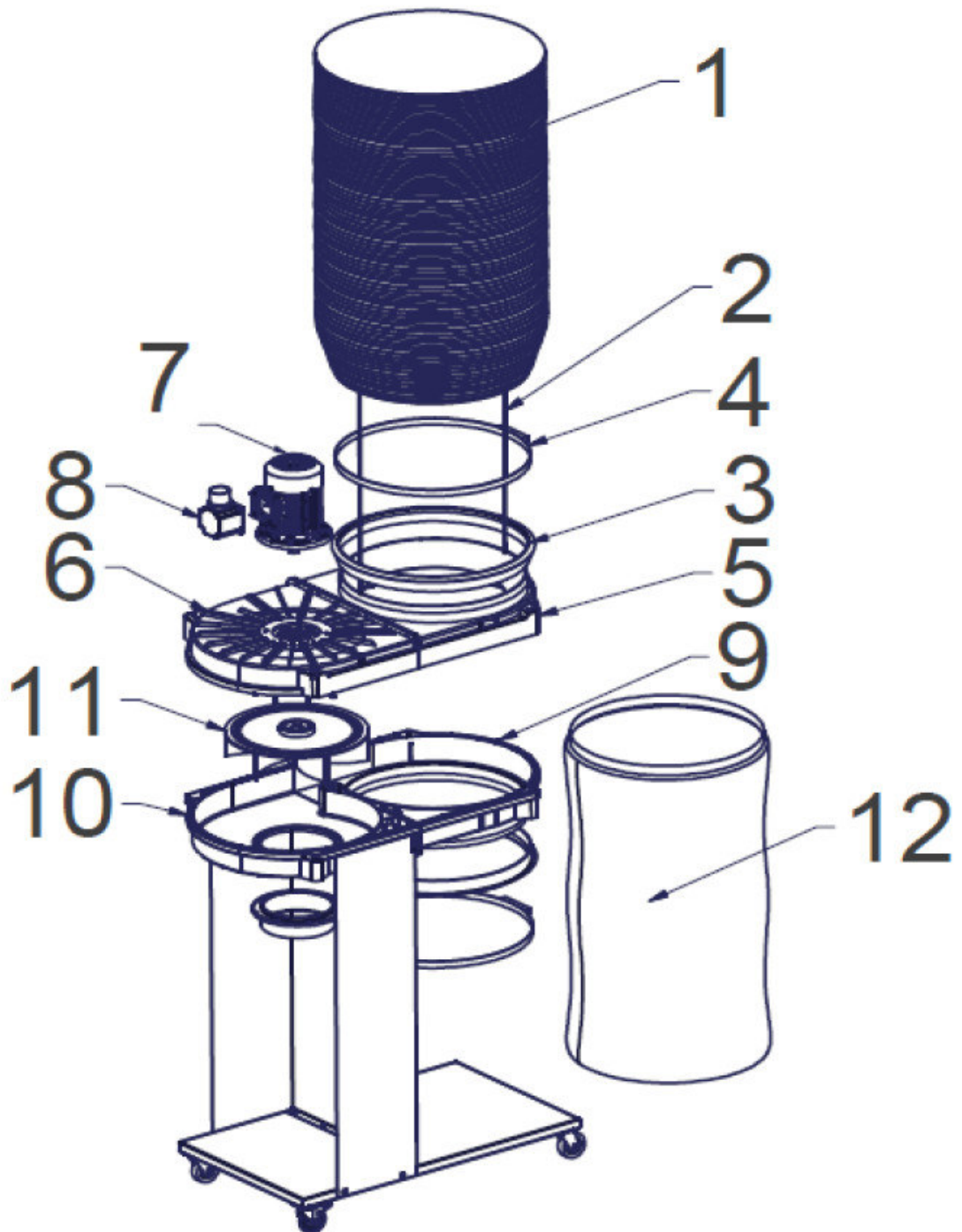
Abb. 15: Ersatzteilzeichnung
