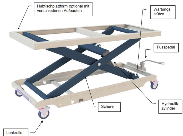
Abb. 4: Gerätebeschreibung HT 600
