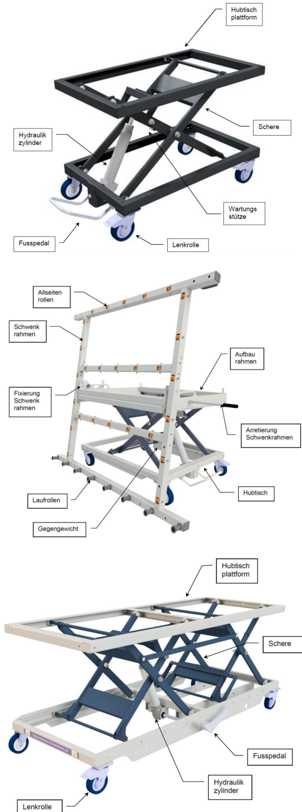
Abb. 3: Gerätebeschreibung HT 300 S und HT 300 M (oben), HT 300 M PSR (Mitte), HT 300 L (unten)
