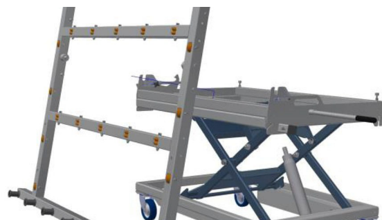
Abb. 5: Abbau der Plattformschwenkeinrichtung
