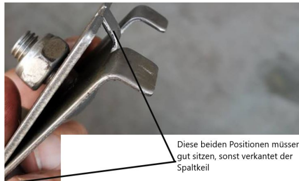
Abb. 20: Spaltkeil montieren Teil 2
