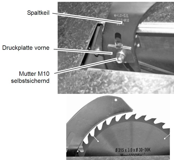
Abb. 22: Montage Spaltkeil
