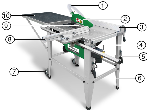
Abb. 5: Tischkreissäge TKS 316 PRO
