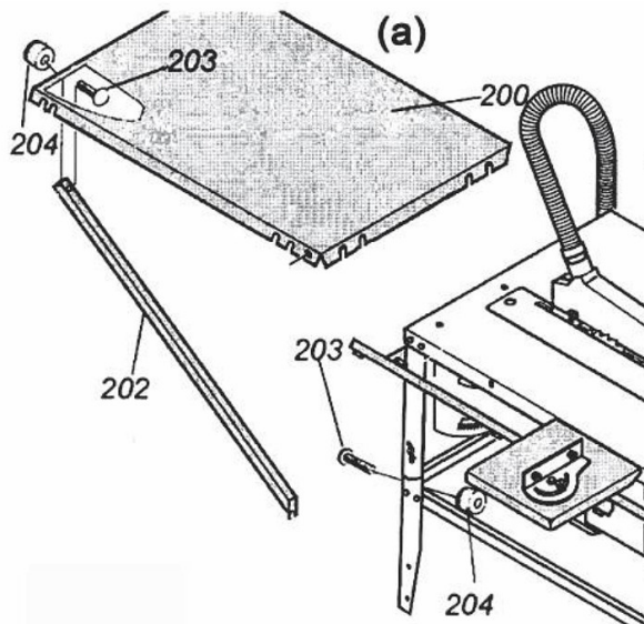
Abb. 25: Tischverlängerung/-erweiterung hinten montieren
