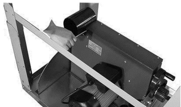
Abb. 9: Absaugstutzen montieren
