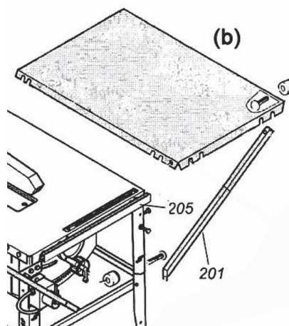
Abb. 26: Tischerweiterung seitlich
