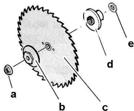
Abb. 17: Sägeblatt
