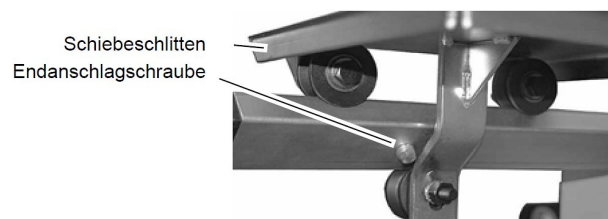
Abb. 14: Montage Laufschiene und Schiebeschlitten
