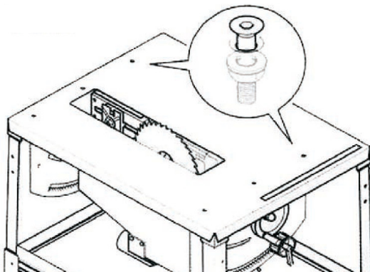
Abb. 18: Sägeblatt ausrichten
