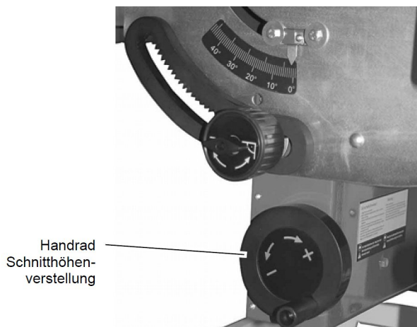
Abb. 29: Schnitthöhe einstellen
