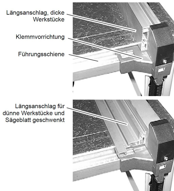
Abb. 31: Sägebetrieb mit Längsanschlag
