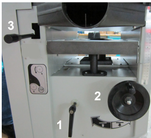
Abb. 10: Höheneinstellung Dickenhobeltisch
