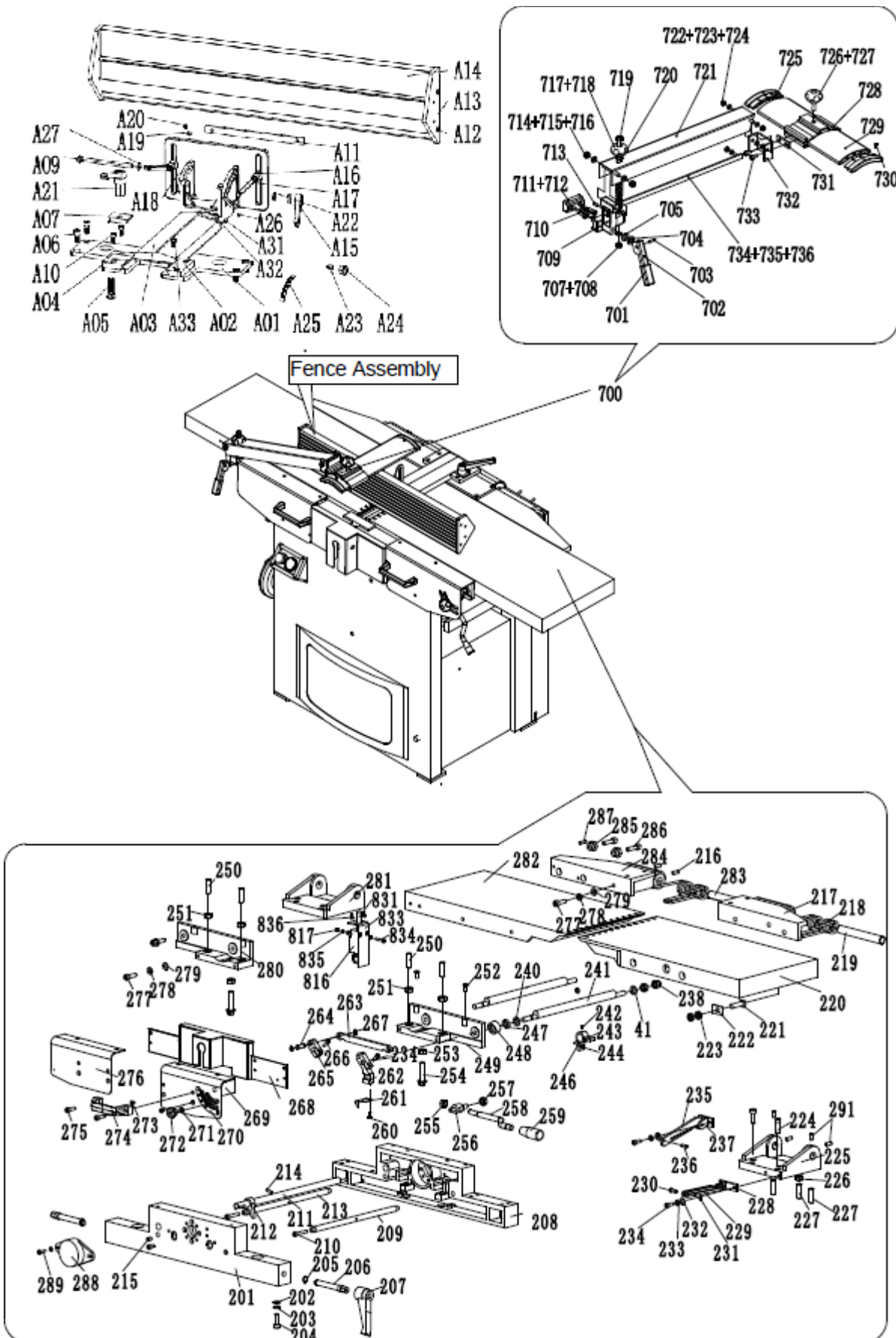
Abb. 27: Ersatzteilzeichnung 2
