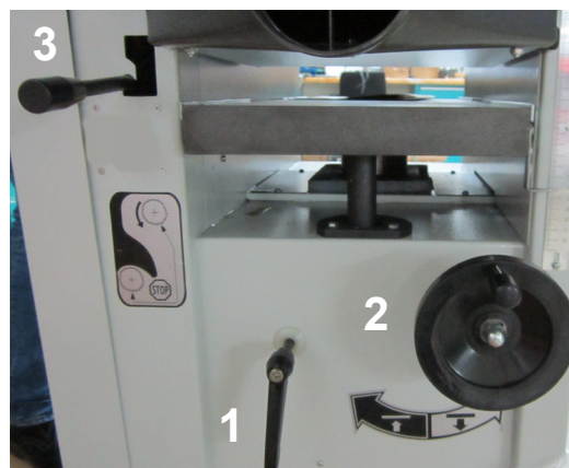
Abb. 19: Höheneinstellung Dickenhobeltisch
