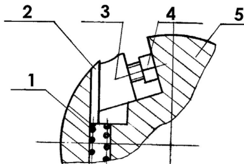
Abb. 11: Messer wechseln
