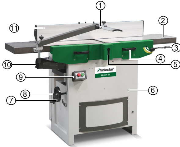
Abb. 4: Abricht- und Dickenhobelmaschine ADH 31-4 C
