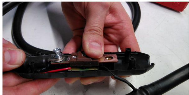
Abb. 16: Polung nicht vertauschen
