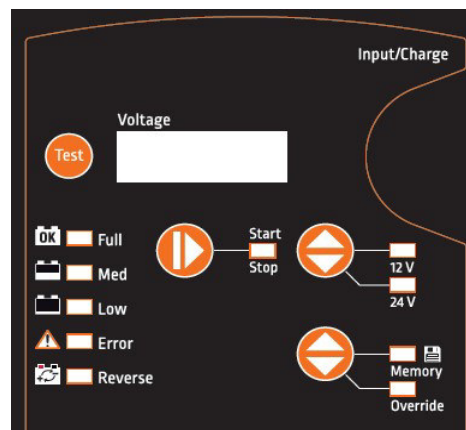
Abb. 8: Bedienfeld SB 202 MS
