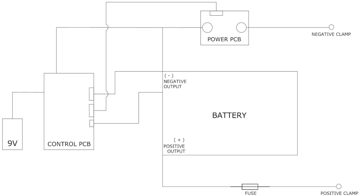
Abb. 26: Elektro-Schaltplan SB 201 MS
