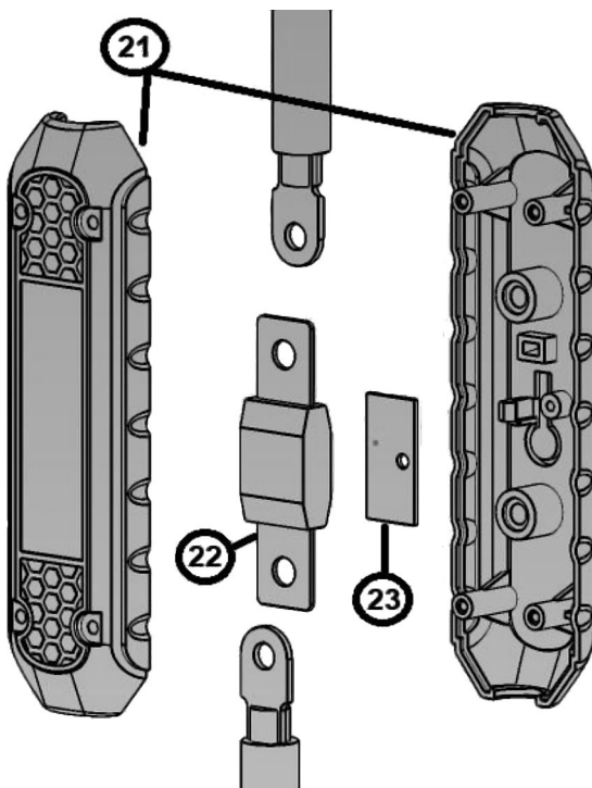
Abb. 25: Ersatzteilzeichnung SB 250, SB 500
