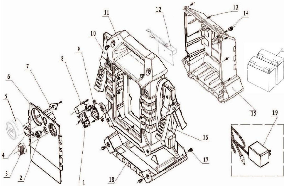
Abb. 24: Ersatzteilzeichnung SB 500
