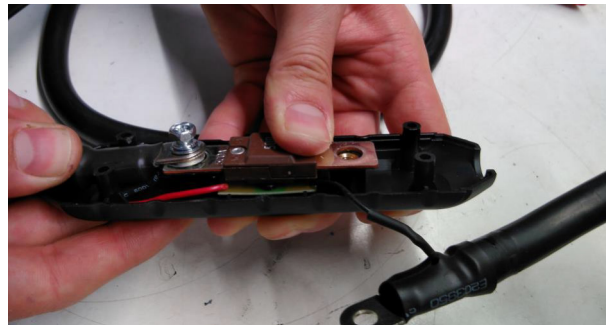
Abb. 15: Neue Sicherung einbauen
