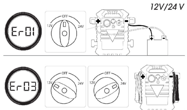
Abb. 10: Fehlerbehebung SB 500
