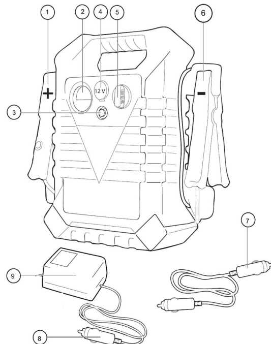
Abb. 3: Startgerät SB 500
