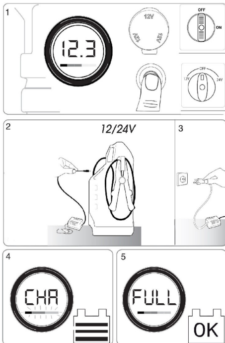
Abb. 9: Ladeschritte
