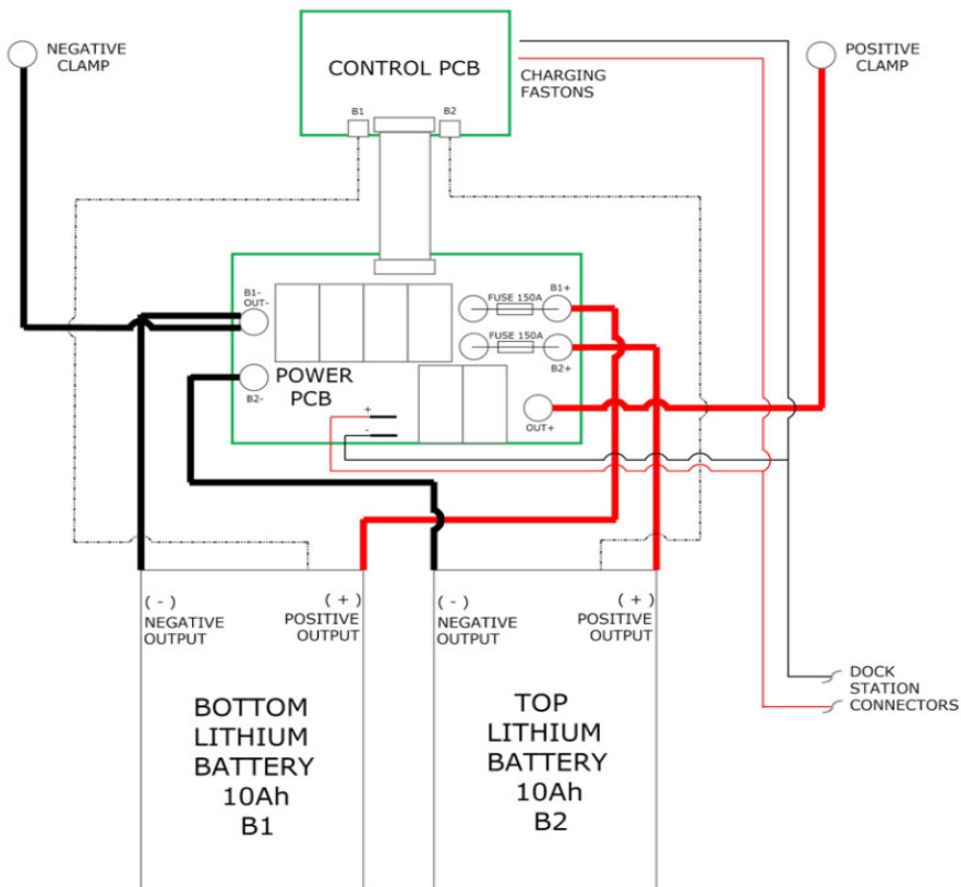
Abb. 27: Elektro-Schaltplan SB 202
