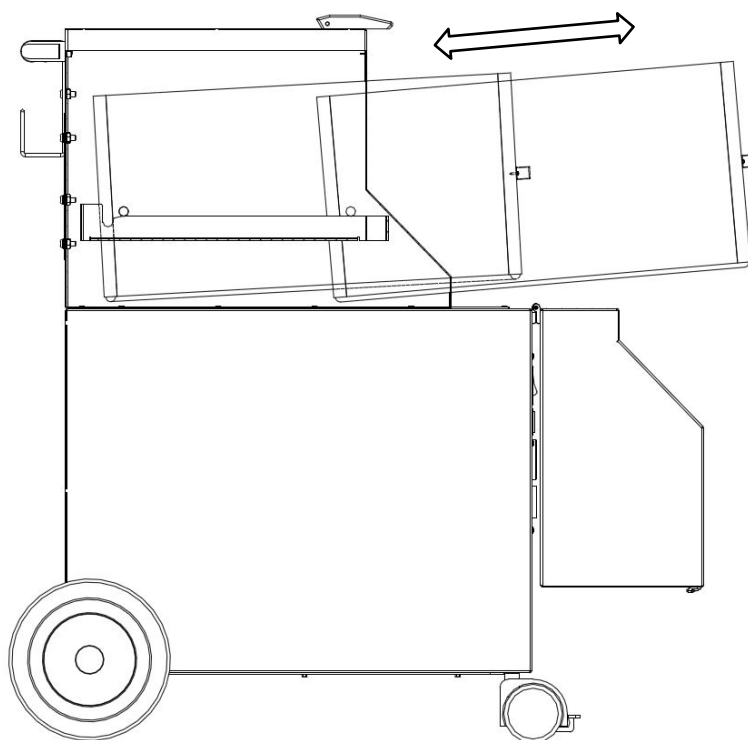
Abbildung 6, Filterwechsel
