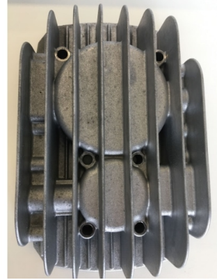
Zylinderkopf (003)
