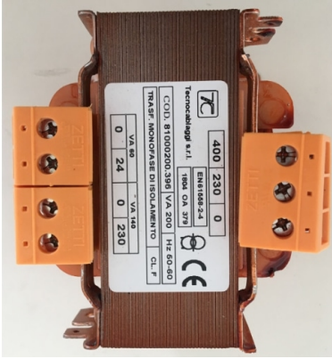
Transformator 400 V auf 230/24 V (TC1)
