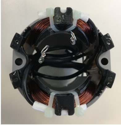
Stator 230V Nr. 35
