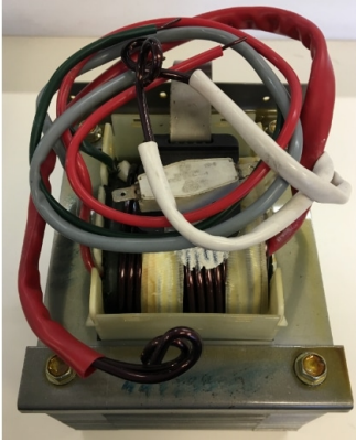
Haupttrafo 12/24 V 230V
