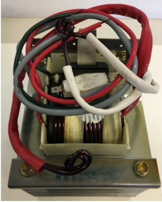
Haupttrafo 12/24 V 230 V
