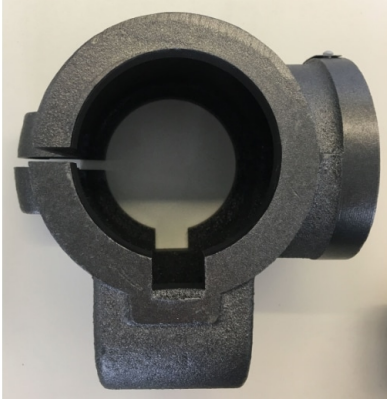
GuÃ?halterung (SÃ?ule) (Nr. 17)
