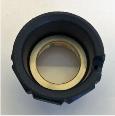
Anschlußmutter (maschinenseitig), Nr. 58 (500.0213)
